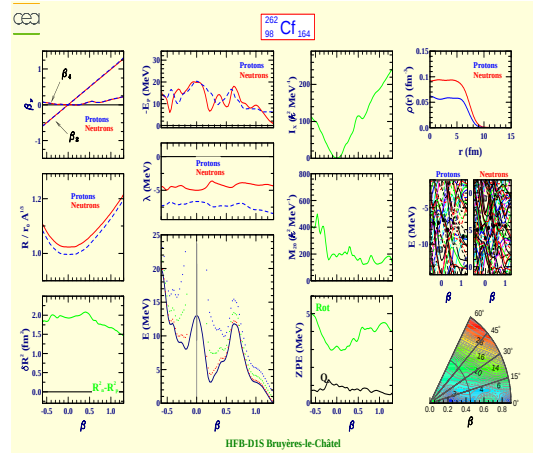
Californium 262 (Z=98, N=164)
