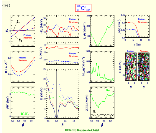
Californium 285 (Z=98, N=187)
