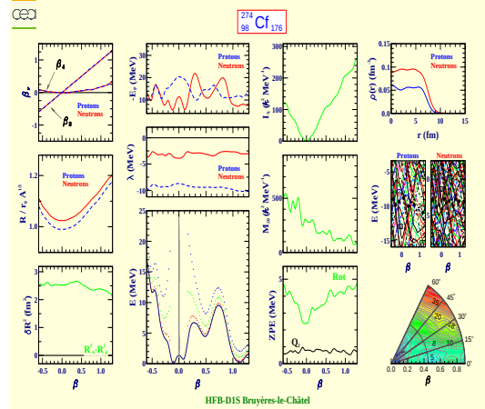
Californium 274 (Z=98, N=176)
