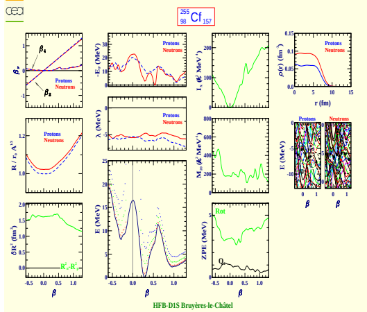
Californium 255 (Z=98, N=157)
