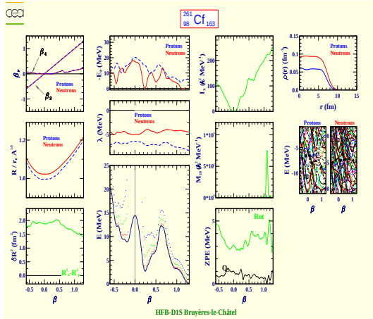
Californium 261 (Z=98, N=163)
