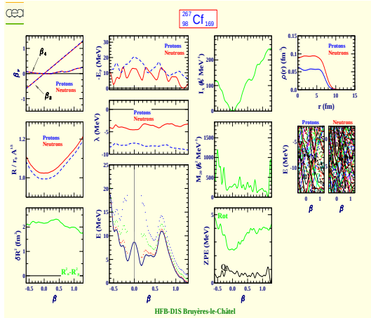
Californium 267 (Z=98, N=169)
