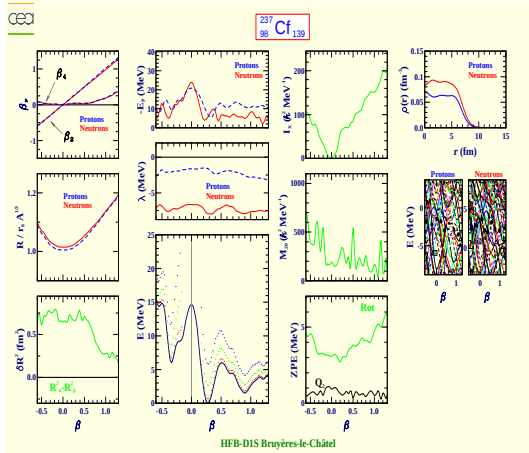
Californium 237 (Z=98, N=139)
