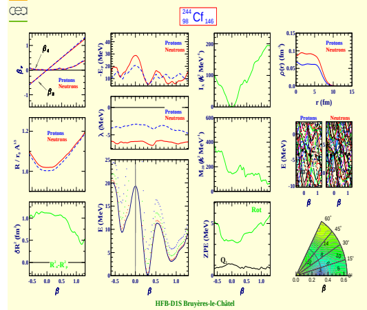
Californium 244 (Z=98, N=146)
