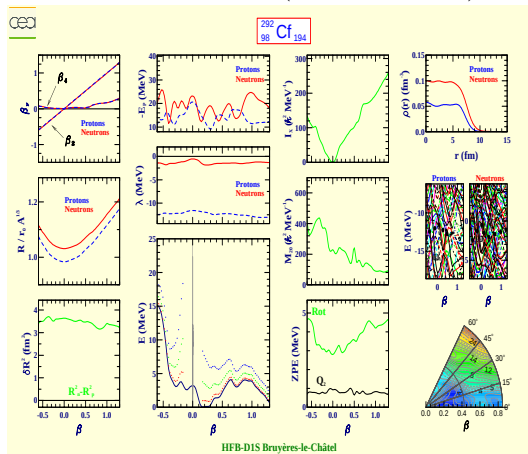
Californium 292 (Z=98, N=194)
