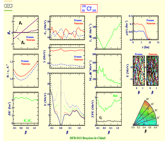
Californium 286 (Z=98, N=188)
