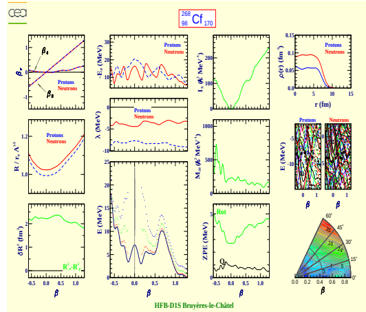
Californium 268 (Z=98, N=170)
