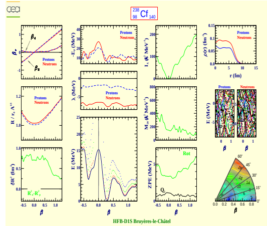
Californium 238 (Z=98, N=140)
