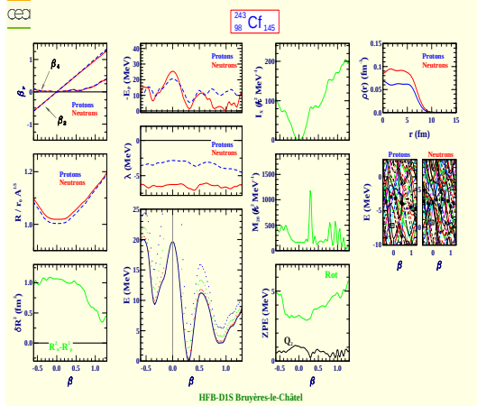
Californium 243 (Z=98, N=145)
