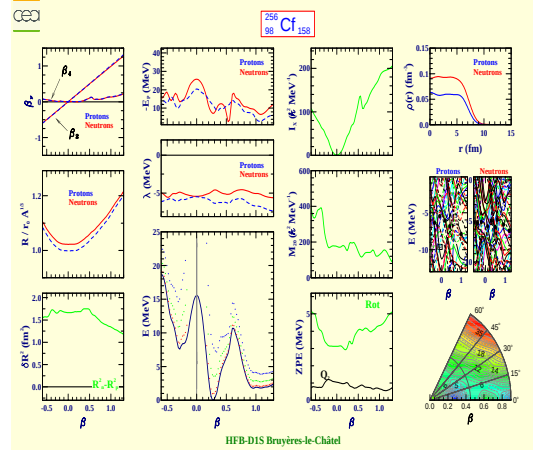
Californium 256 (Z=98, N=158)
