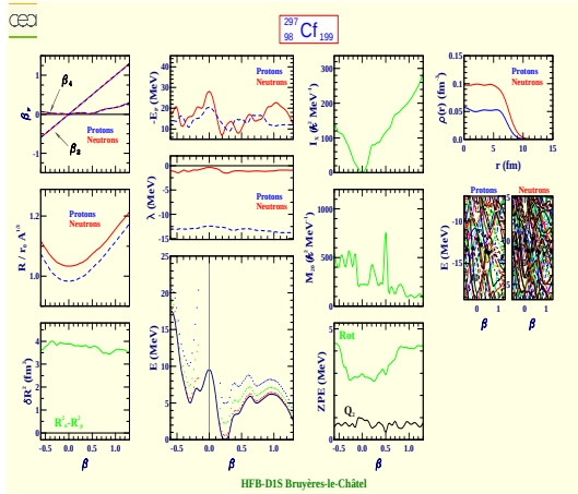
Californium 297 (Z=98, N=199)
