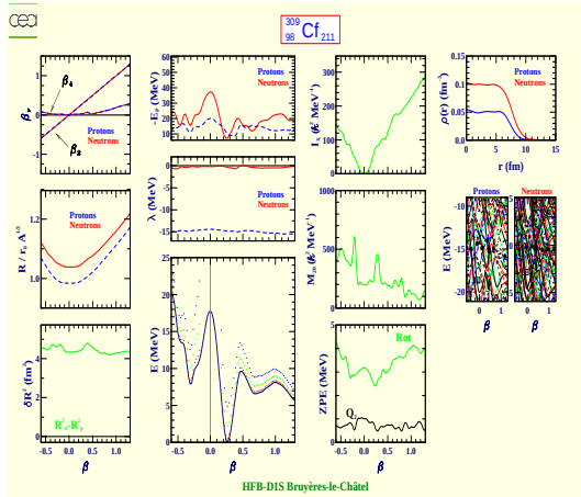
Californium 309 (Z=98, N=211)
