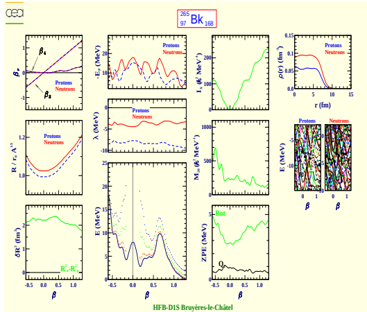
Berkelium 265 (Z=97, N=168)
