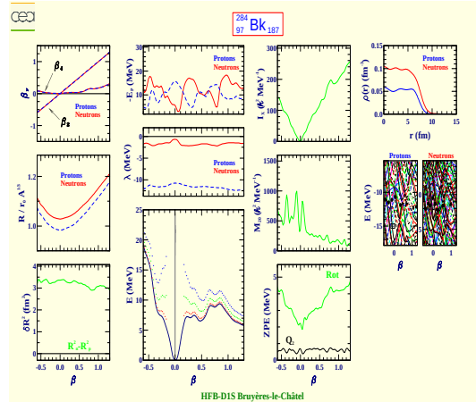
Berkelium 284 (Z=97, N=187)
