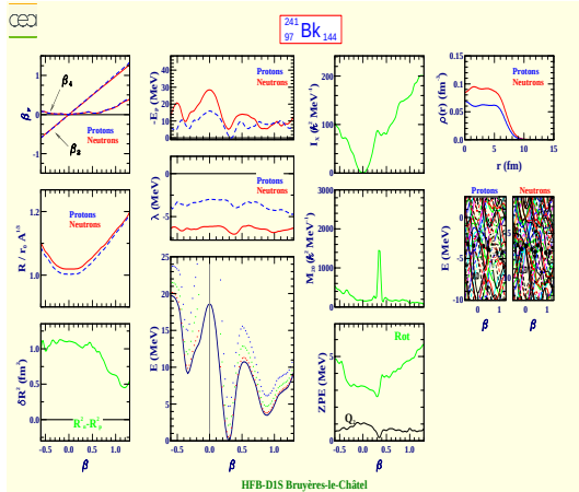
Berkelium 241 (Z=97, N=144)
