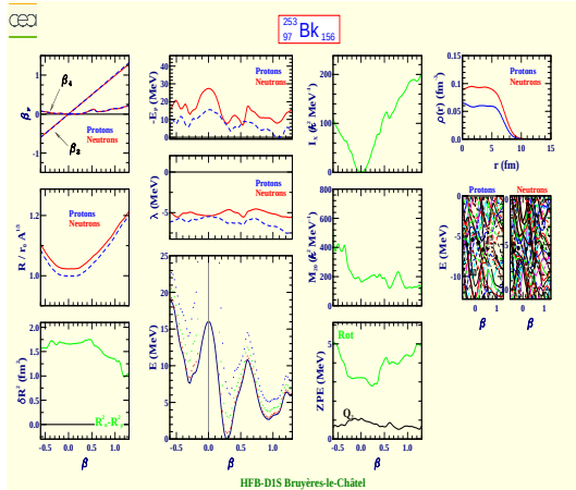
Berkelium 253 (Z=97, N=156)
