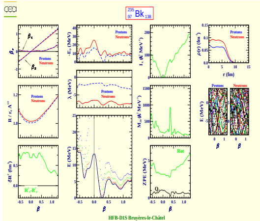
Berkelium 235 (Z=97, N=138)
