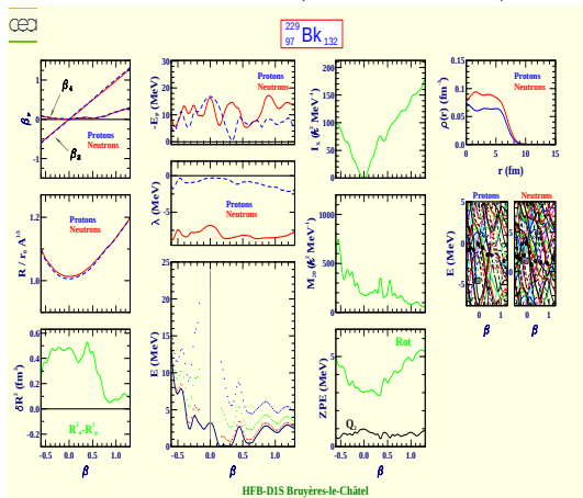
Berkelium 229 (Z=97, N=132)
