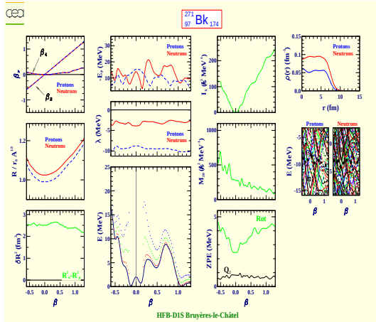
Berkelium 271 (Z=97, N=174)
