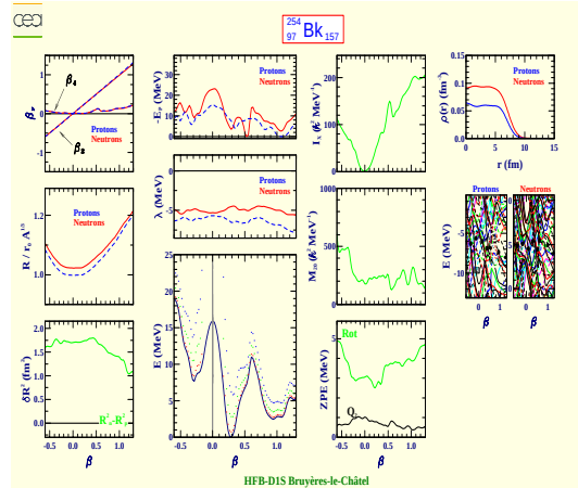
Berkelium 254 (Z=97, N=157)
