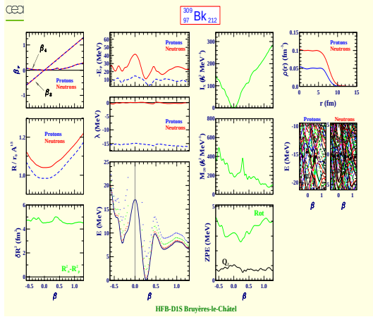
Berkelium 309 (Z=97, N=212)
