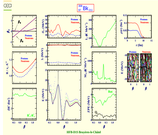
Berkelium 308 (Z=97, N=211)
