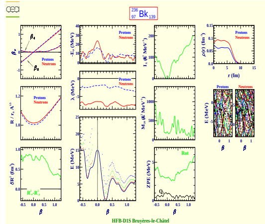
Berkelium 236 (Z=97, N=139)
