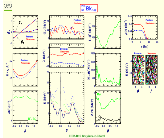
Berkelium 266 (Z=97, N=169)
