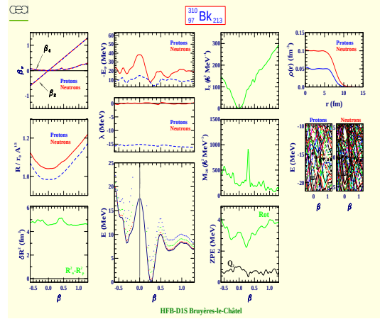
Berkelium 310 (Z=97, N=213)
