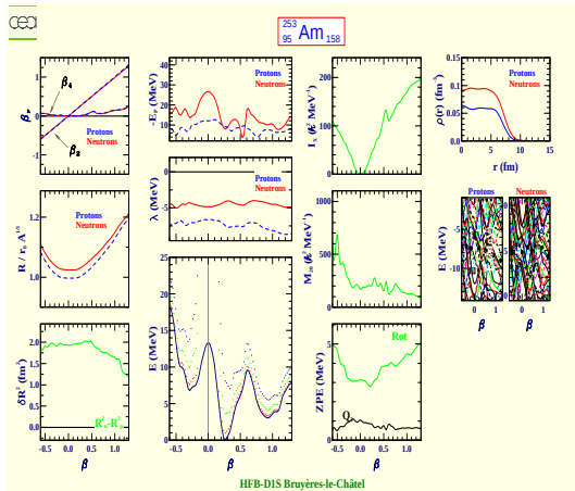
Américium 253 (Z=95, N=158)
