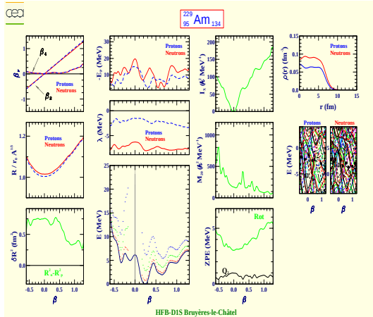
Américium 229 (Z=95, N=134)
