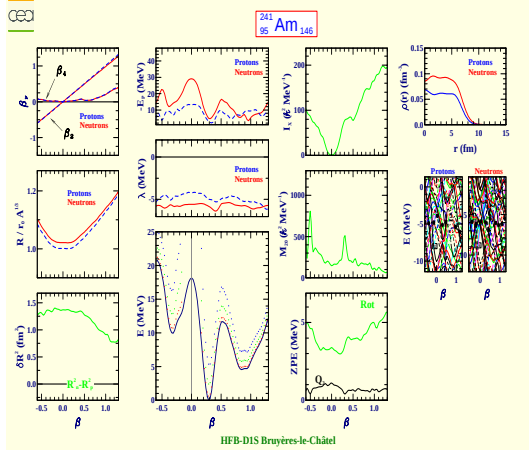
Américium 241 (Z=95, N=146)
