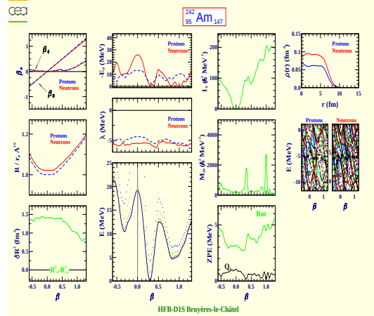
Américium 242 (Z=95, N=147)
