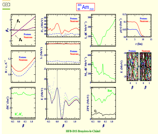
Américium 305 (Z=95, N=210)
