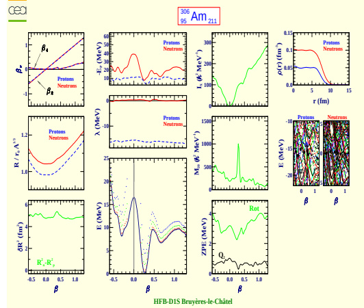
Américium 306 (Z=95, N=211)
