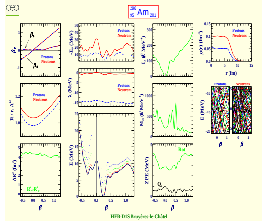
Américium 296 (Z=95, N=201)
