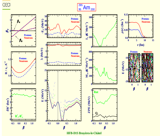
Américium 295 (Z=95, N=200)
