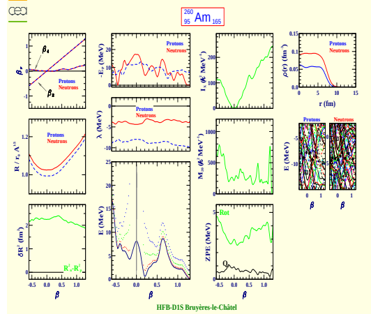
Américium 260 (Z=95, N=165)
