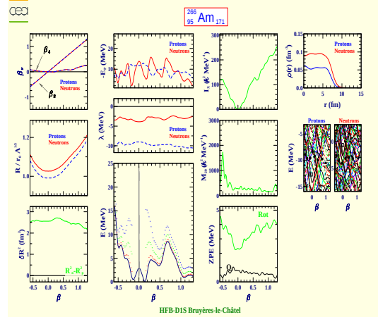
Américium 266 (Z=95, N=171)
