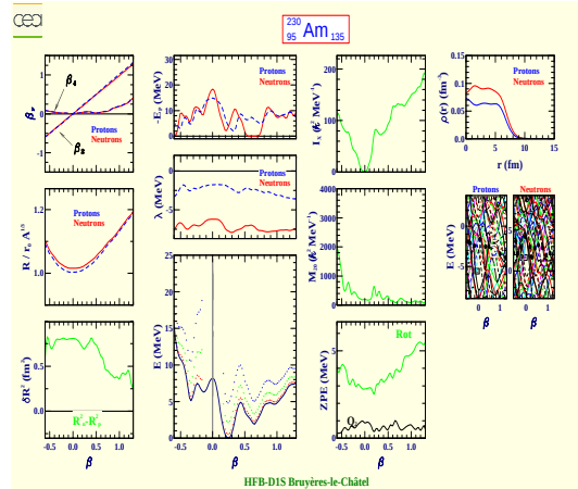
Américium 230 (Z=95, N=135)
