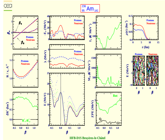
Américium 236 (Z=95, N=141)
