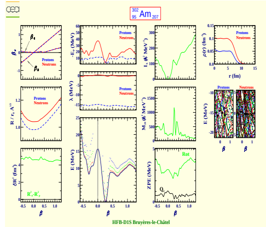
Américium 302 (Z=95, N=207)
