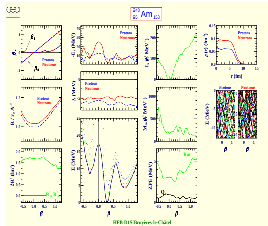
Américium 248 (Z=95, N=153)
