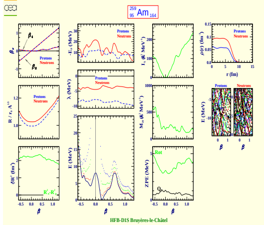
Américium 259 (Z=95, N=164)
