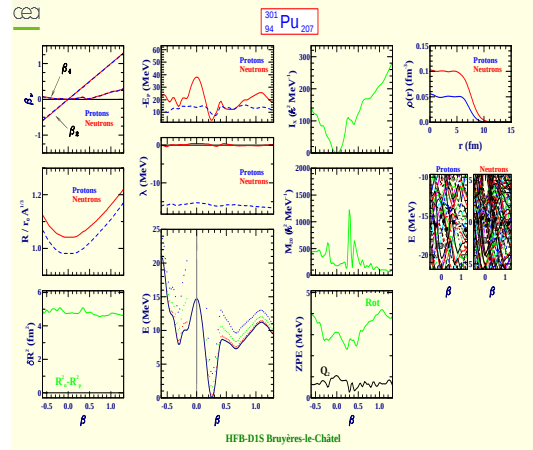
Plutonium 301 (Z=94, N=207)
