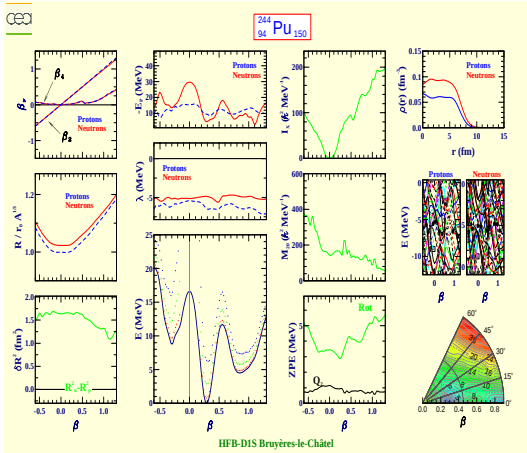
Plutonium 244 (Z=94, N=150)
