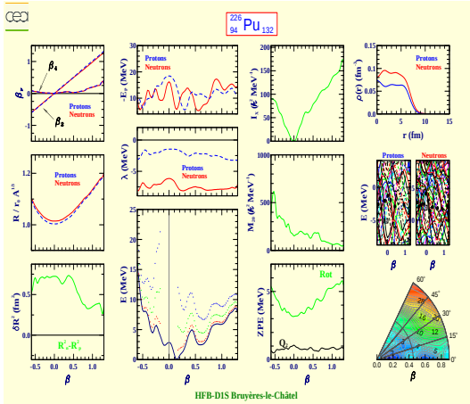
Plutonium 226 (Z=94, N=132)
