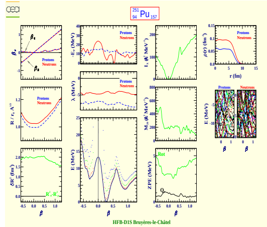
Plutonium 251 (Z=94, N=157)
