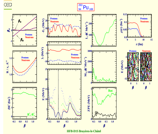
Plutonium 263 (Z=94, N=169)
