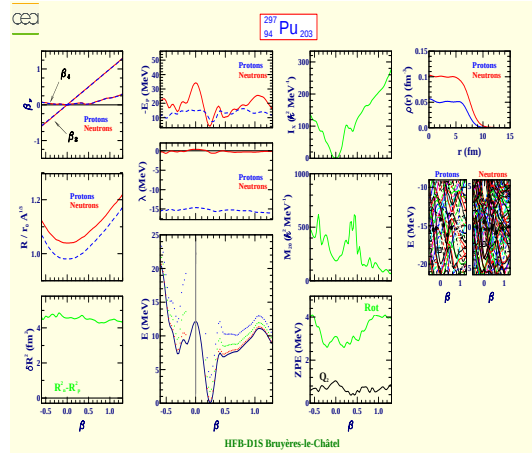
Plutonium 297 (Z=94, N=203)
