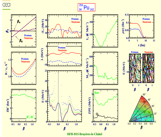
Plutonium 256 (Z=94, N=162)
