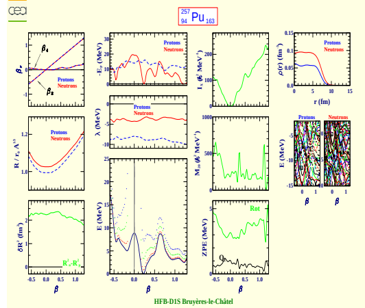
Plutonium 257 (Z=94, N=163)
