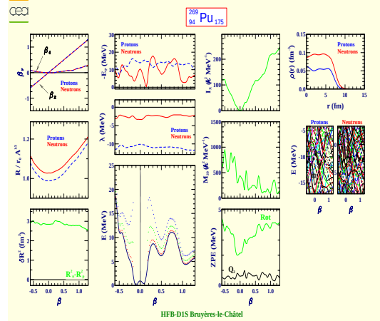
Plutonium 269 (Z=94, N=175)
