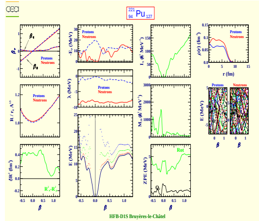
Plutonium 221 (Z=94, N=127)
