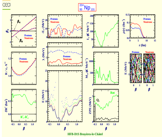
Neptunium 224 (Z=93, N=131)
