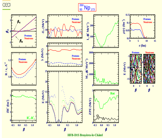
Neptunium 266 (Z=93, N=173)
