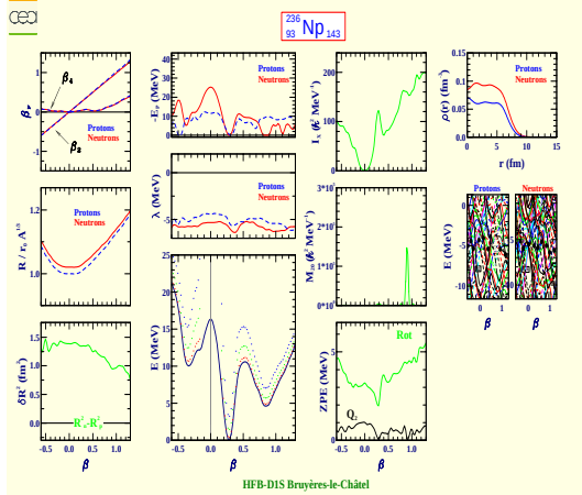
Neptunium 236 (Z=93, N=143)
