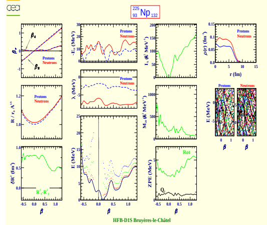
Neptunium 225 (Z=93, N=132)
