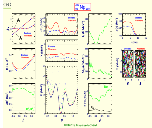
Neptunium 243 (Z=93, N=150)
