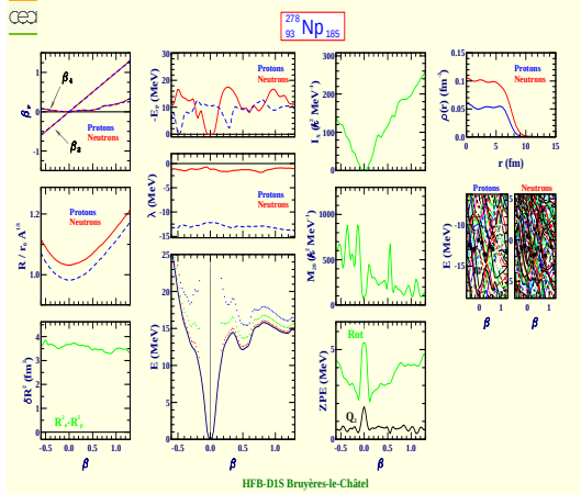
Neptunium 278 (Z=93, N=185)
