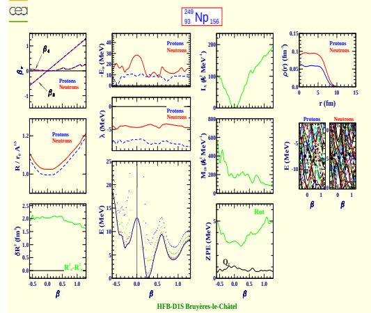
Neptunium 249 (Z=93, N=156)
