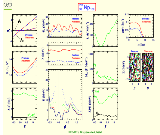
Neptunium 261 (Z=93, N=168)
