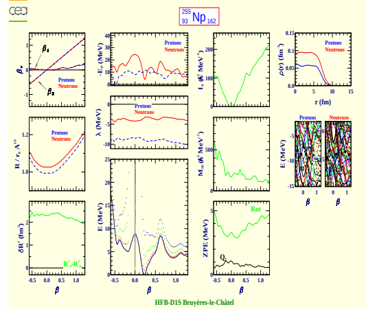
Neptunium 255 (Z=93, N=162)
