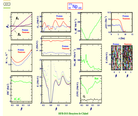
Neptunium 273 (Z=93, N=180)
