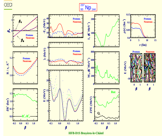
Neptunium 237 (Z=93, N=144)
