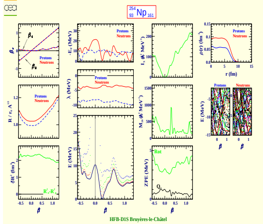
Neptunium 254 (Z=93, N=161)
