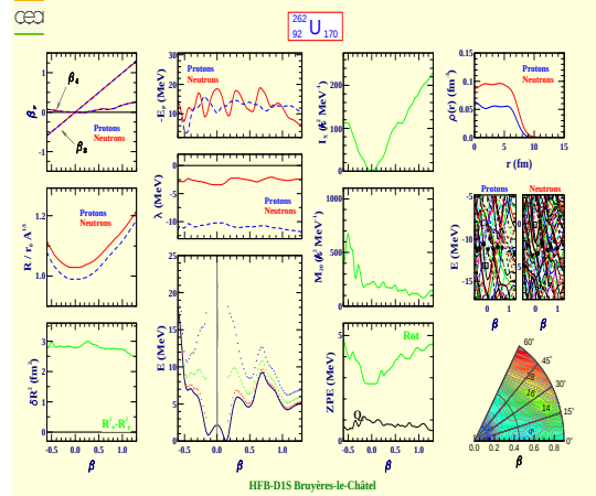
Uranium 262 (Z=92, N=170)
