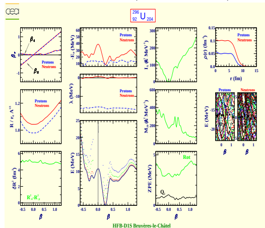
Uranium 296 (Z=92, N=204)
