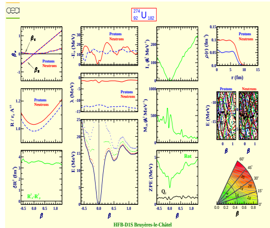
Uranium 274 (Z=92, N=182)
