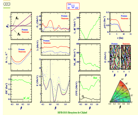
Uranium 244 (Z=92, N=152)
