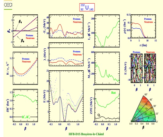
Uranium 232 (Z=92, N=140)
