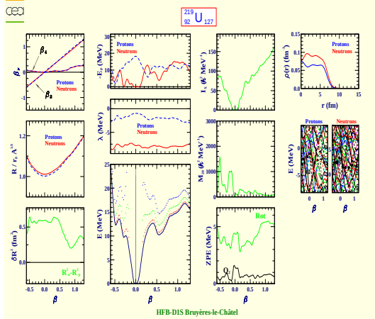
Uranium 219 (Z=92, N=127)
