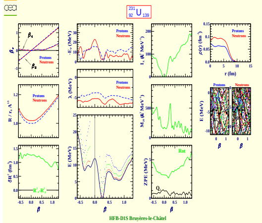
Uranium 231 (Z=92, N=139)
