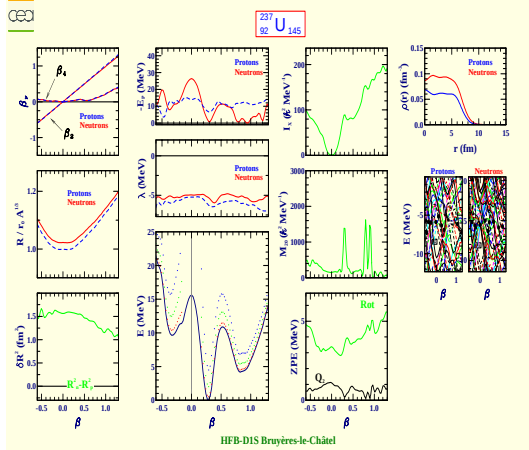
Uranium 237 (Z=92, N=145)
