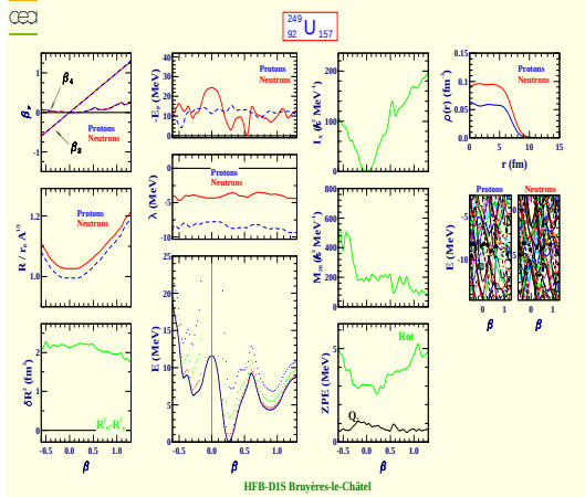
Uranium 249 (Z=92, N=157)
