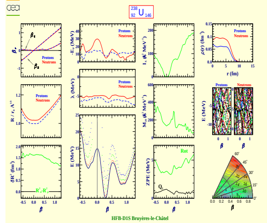
Uranium 238 (Z=92, N=146)
