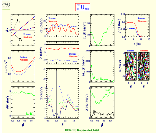
Uranium 261 (Z=92, N=169)
