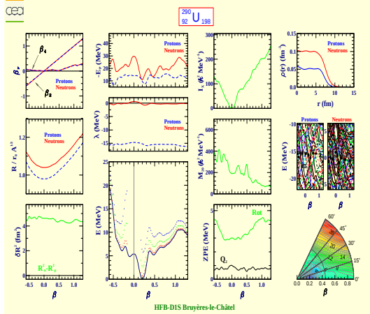
Uranium 290 (Z=92, N=198)
