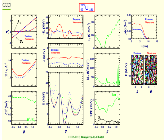
Uranium 243 (Z=92, N=151)
