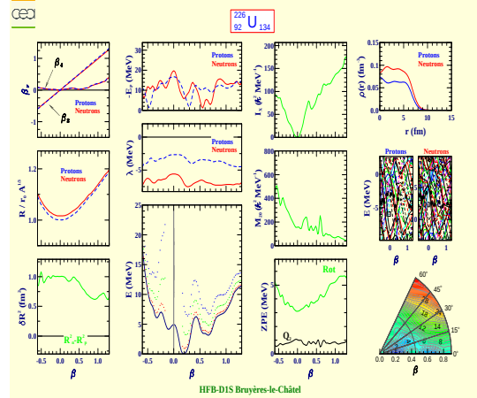
Uranium 226 (Z=92, N=134)
