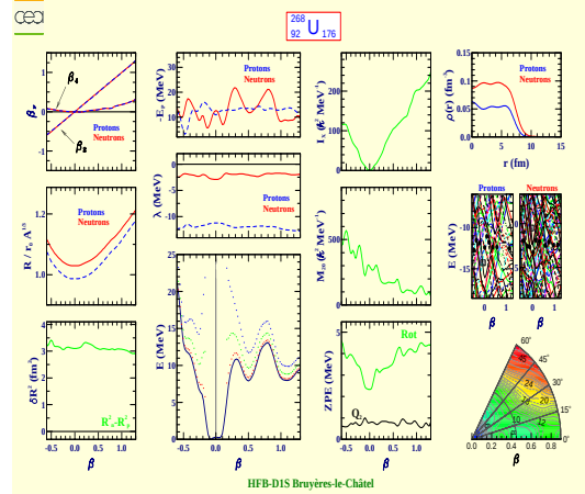
Uranium 268 (Z=92, N=176)
