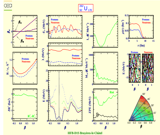
Uranium 262 (Z=92, N=170)
