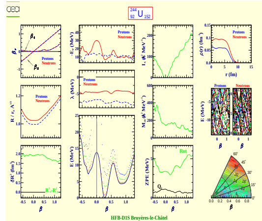
Uranium 244 (Z=92, N=152)
