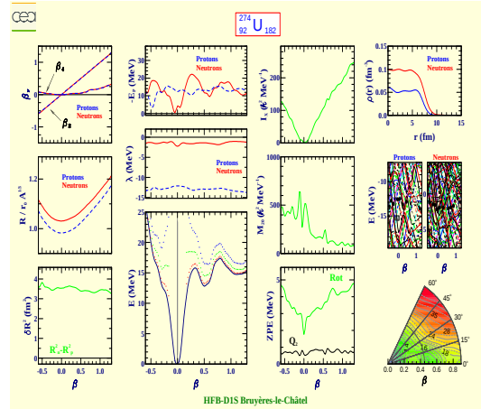
Uranium 274 (Z=92, N=182)
