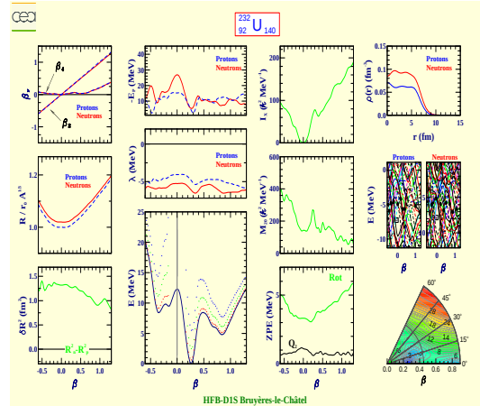
Uranium 232 (Z=92, N=140)
