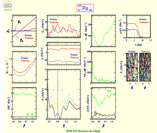
Protactinium 260 (Z=91, N=169)
