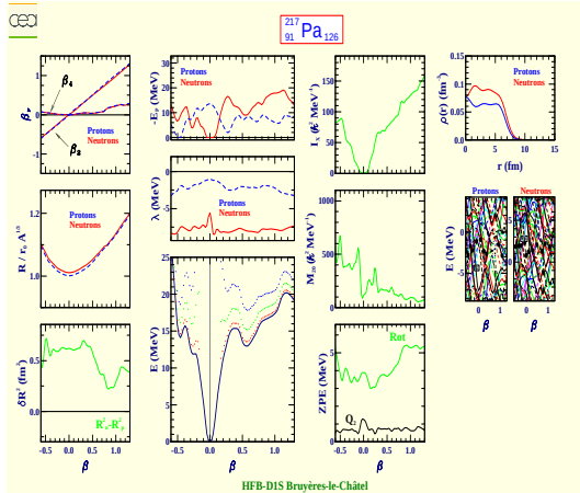
Protactinium 217 (Z=91, N=126)
