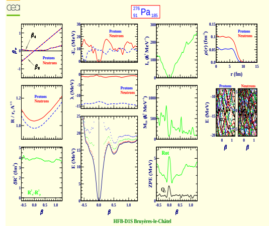
Protactinium 276 (Z=91, N=185)
