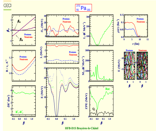
Protactinium 272 (Z=91, N=181)
