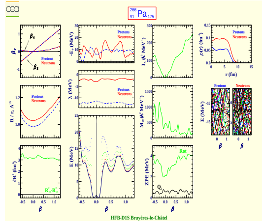
Protactinium 266 (Z=91, N=175)
