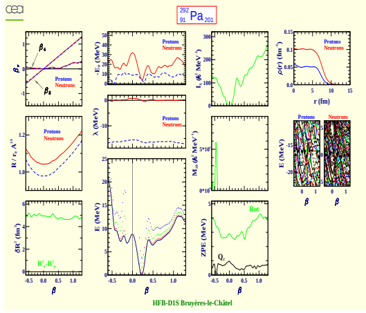
Protactinium 292 (Z=91, N=201)
