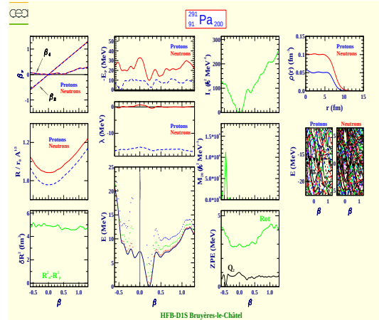
Protactinium 291 (Z=91, N=200)
