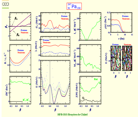
Protactinium 247 (Z=91, N=156)
