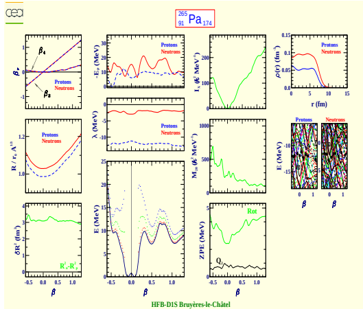
Protactinium 265 (Z=91, N=174)
