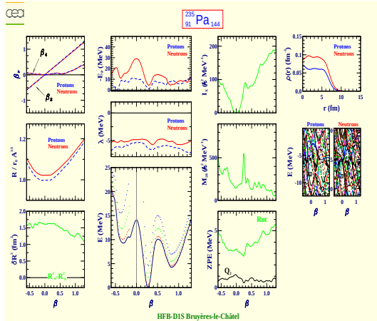
Protactinium 235 (Z=91, N=144)
