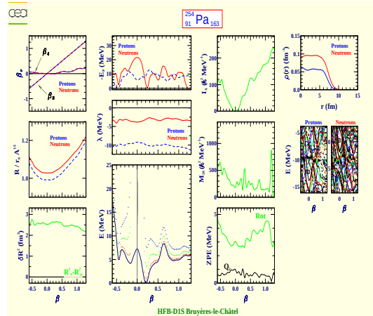
Protactinium 254 (Z=91, N=163)
