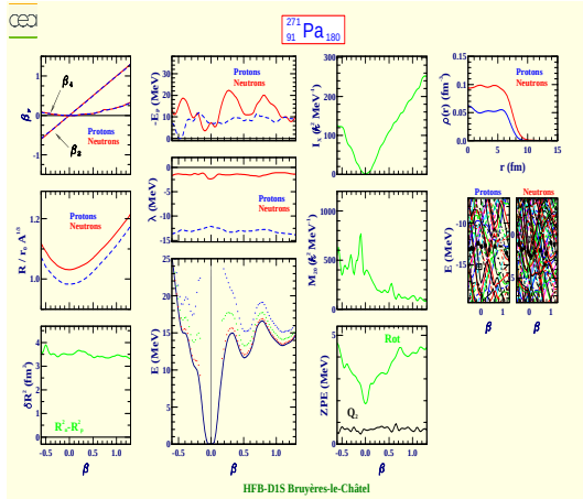
Protactinium 271 (Z=91, N=180)
