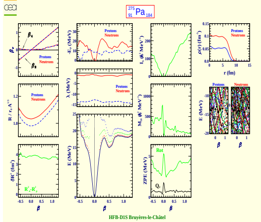
Protactinium 275 (Z=91, N=184)
