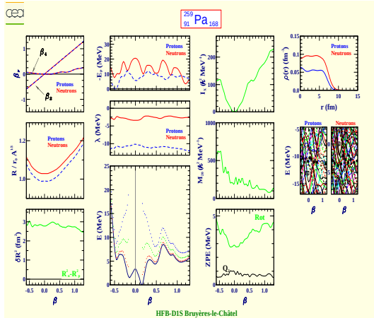
Protactinium 259 (Z=91, N=168)
