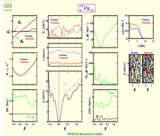
Protactinium 218 (Z=91, N=127)
