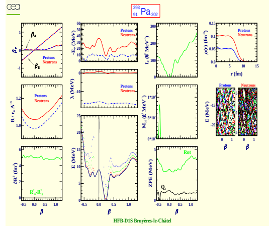
Protactinium 293 (Z=91, N=202)
