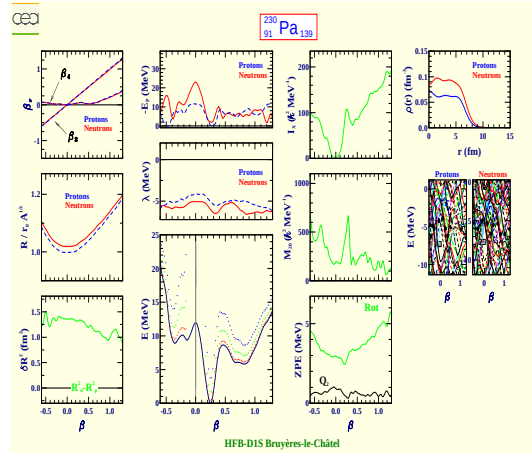
Protactinium 230 (Z=91, N=139)
