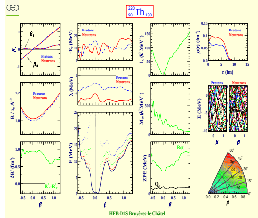
Thorium 220 (Z=90, N=130)
