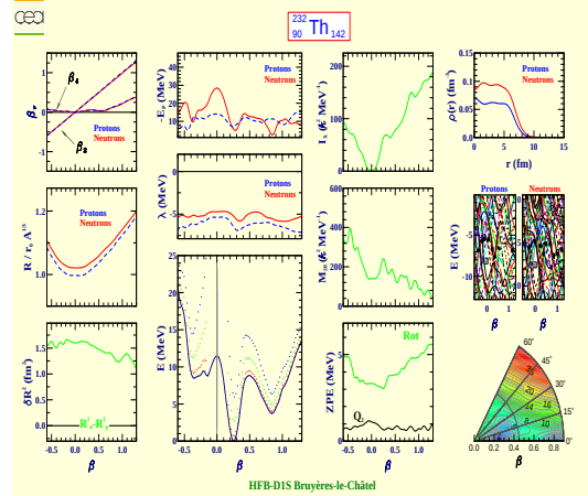
Thorium 232 (Z=90, N=142)
