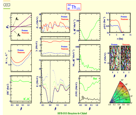
Thorium 262 (Z=90, N=172)
