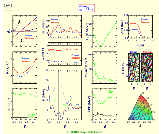
Thorium 256 (Z=90, N=166)
