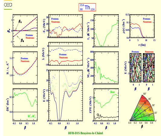
Thorium 214 (Z=90, N=124)
