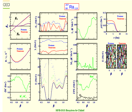
Radium 207 (Z=88, N=119)
