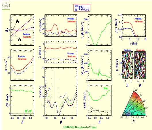
Radium 248 (Z=88, N=160)
