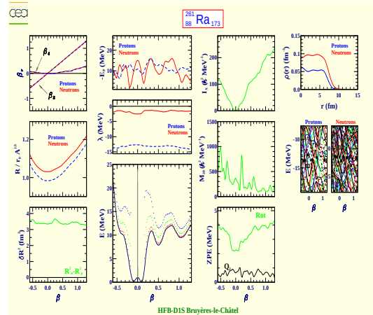
Radium 261 (Z=88, N=173)
