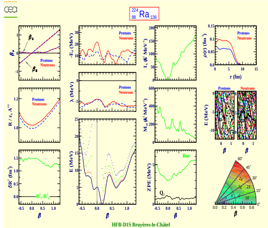
Radium 224 (Z=88, N=136)
