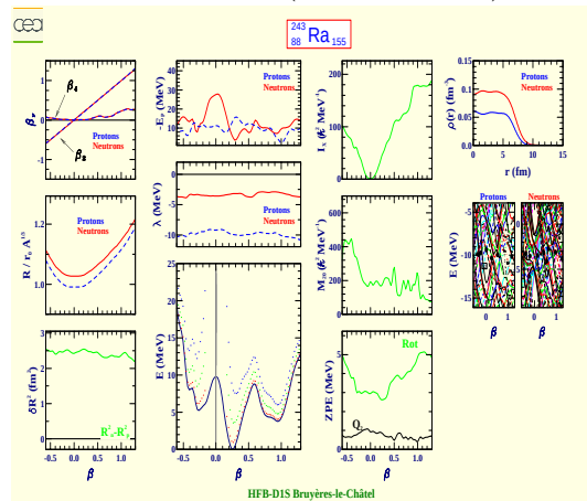
Radium 243 (Z=88, N=155)
