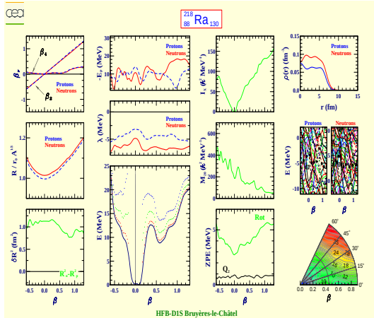
Radium 218 (Z=88, N=130)
