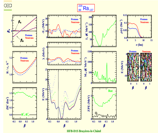
Radium 225 (Z=88, N=137)
