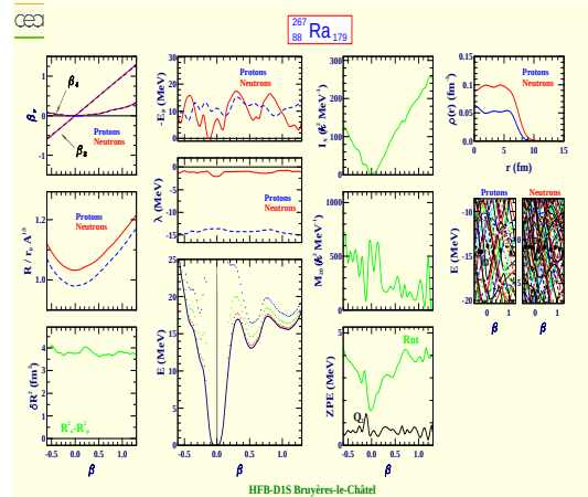
Radium 267 (Z=88, N=179)
