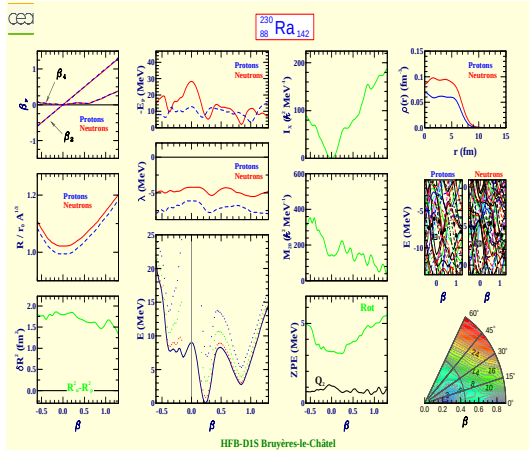
Radium 230 (Z=88, N=142)
