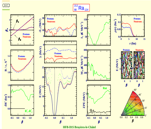
Radium 212 (Z=88, N=124)
