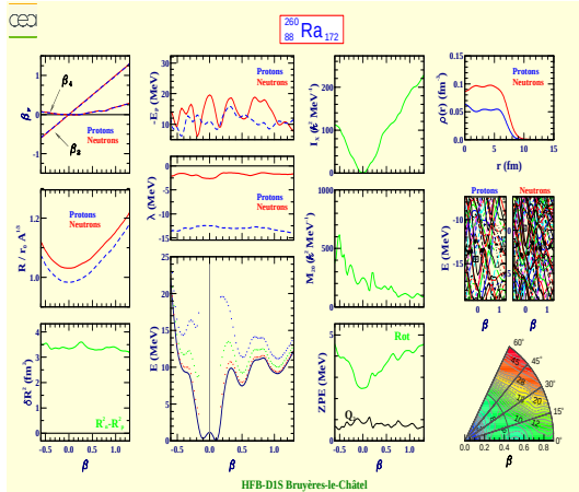
Radium 260 (Z=88, N=172)
