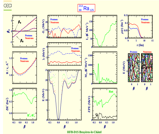
Radium 213 (Z=88, N=125)
