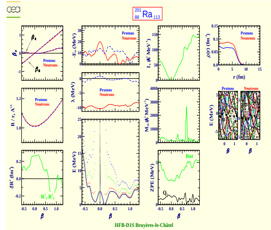
Radium 201 (Z=88, N=113)
