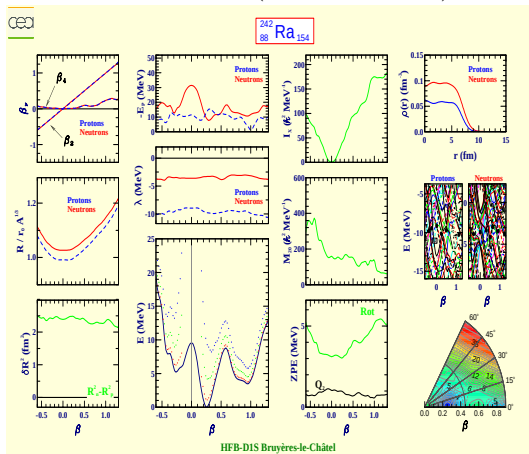
Radium 242 (Z=88, N=154)
