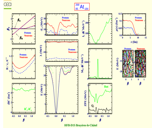
Astatine 269 (Z=85, N=184)
