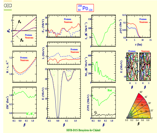
Polonium 208 (Z=84, N=124)
