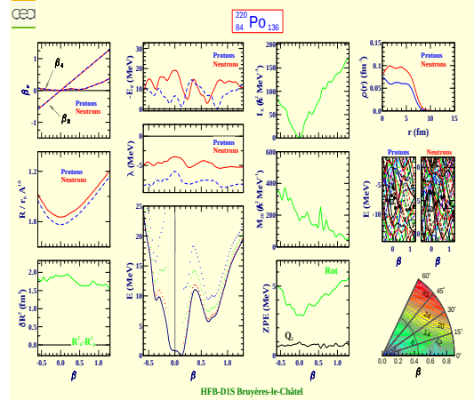
Polonium 220 (Z=84, N=136)
