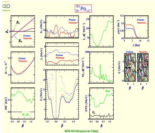
Polonium 201 (Z=84, N=117)
