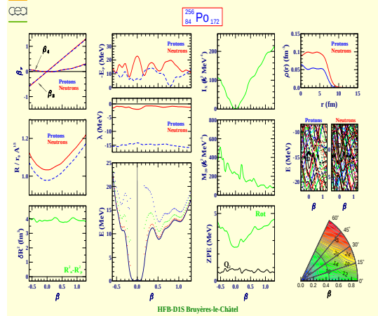
Polonium 256 (Z=84, N=172)
