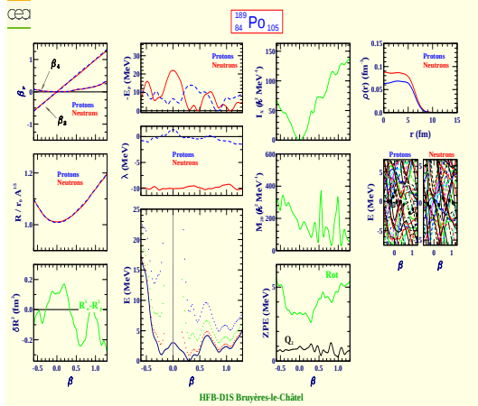
Polonium 189 (Z=84, N=105)
