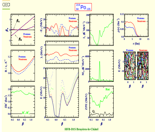
Polonium 219 (Z=84, N=135)
