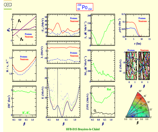
Polonium 238 (Z=84, N=154)
