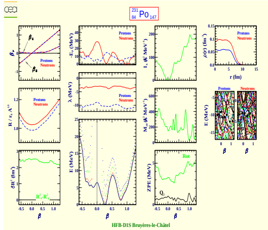
Polonium 231 (Z=84, N=147)
