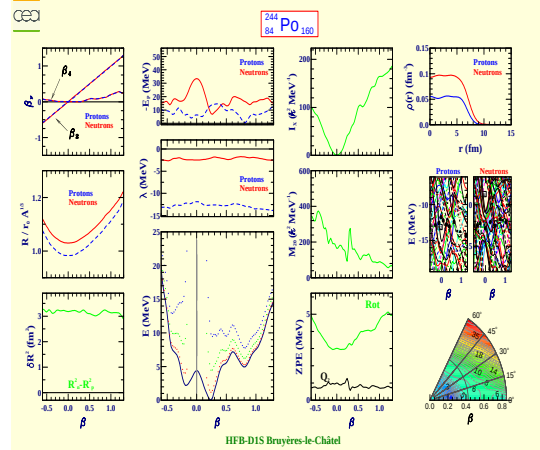
Polonium 244 (Z=84, N=160)
