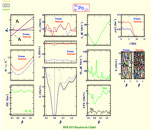
Polonium 261 (Z=84, N=177)
