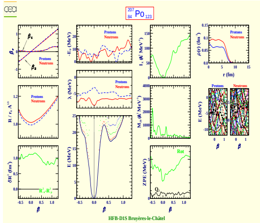
Polonium 207 (Z=84, N=123)
