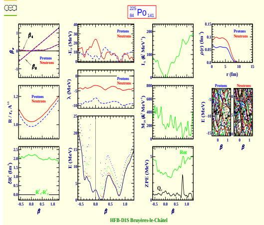
Polonium 225 (Z=84, N=141)
