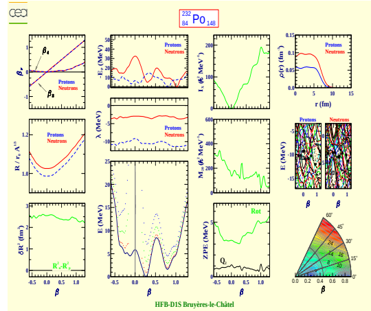
Polonium 232 (Z=84, N=148)
