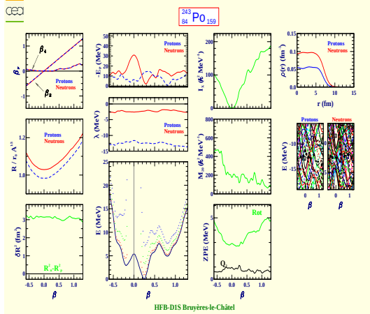
Polonium 243 (Z=84, N=159)
