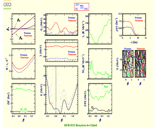
Thallium 227 (Z=81, N=146)
