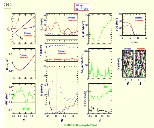
Thallium 185 (Z=81, N=104)
