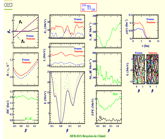
Thallium 215 (Z=81, N=134)
