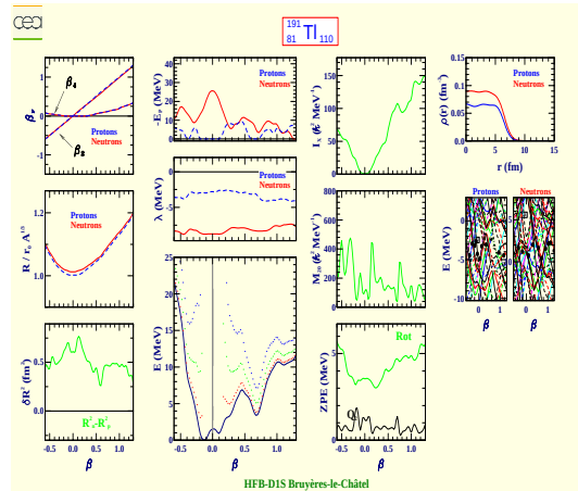
Thallium 191 (Z=81, N=110)
