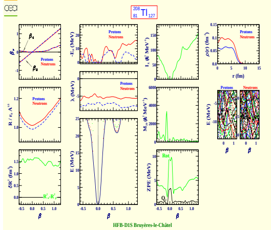
Thallium 208 (Z=81, N=127)
