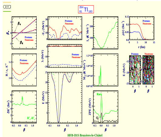
Thallium 264 (Z=81, N=183)
