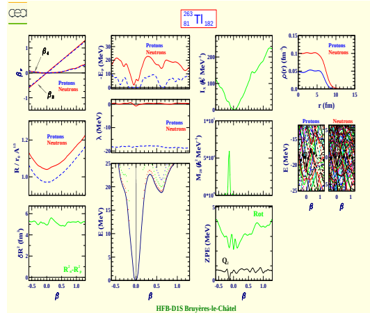
Thallium 263 (Z=81, N=182)
