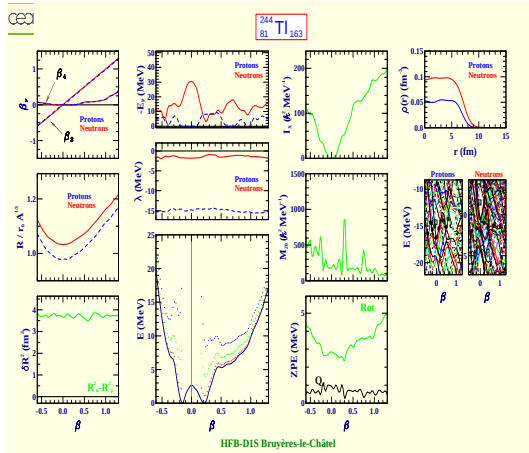
Thallium 244 (Z=81, N=163)
