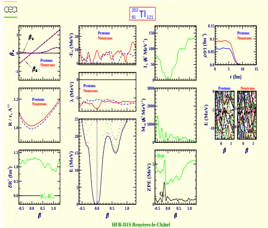
Thallium 202 (Z=81, N=121)
