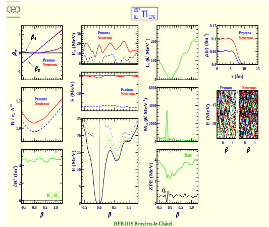
Thallium 257 (Z=81, N=176)
