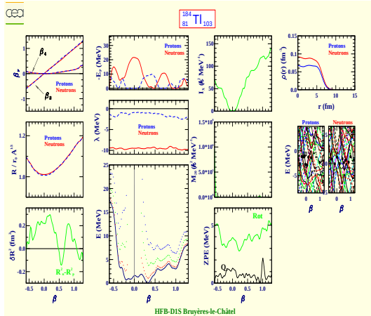
Thallium 184 (Z=81, N=103)
