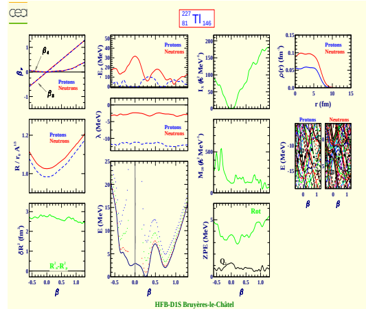
Thallium 227 (Z=81, N=146)
