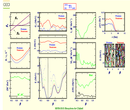
Thallium 221 (Z=81, N=140)
