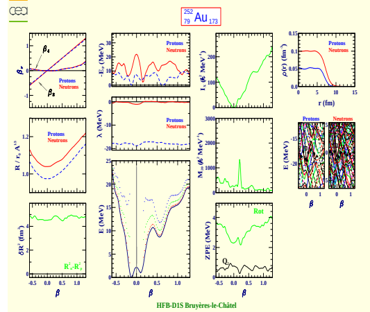
Gold 252 (Z=79, N=173)
