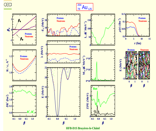
Gold 204 (Z=79, N=125)
