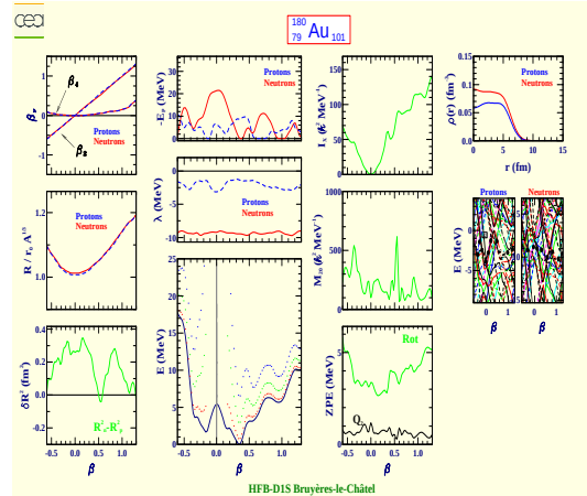
Gold 180 (Z=79, N=101)
