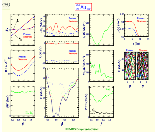
Gold 251 (Z=79, N=172)
