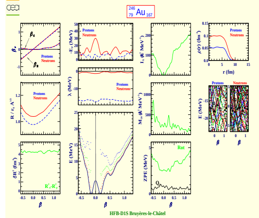
Gold 246 (Z=79, N=167)
