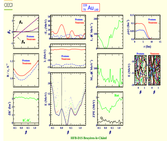
Gold 228 (Z=79, N=149)
