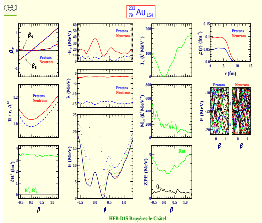
Gold 233 (Z=79, N=154)
