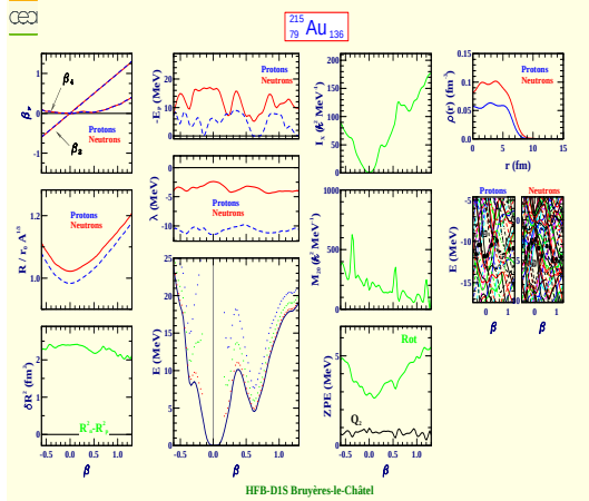
Gold 215 (Z=79, N=136)
