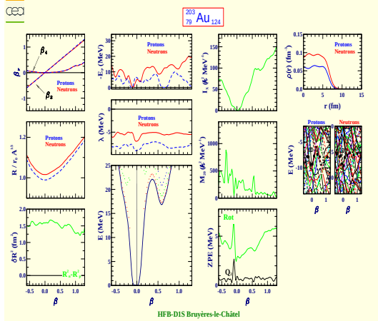
Gold 203 (Z=79, N=124)
