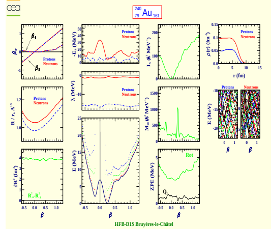
Gold 240 (Z=79, N=161)
