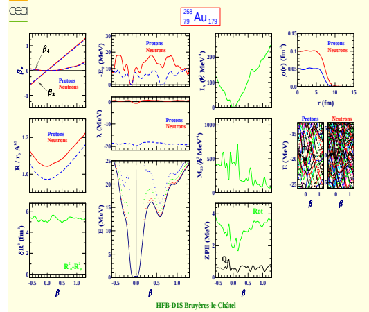
Gold 258 (Z=79, N=179)
