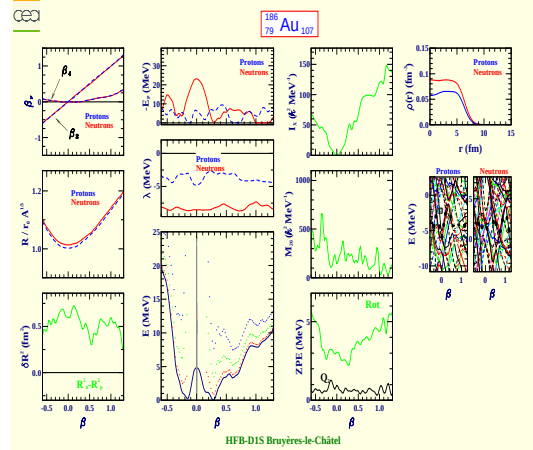
Gold 186 (Z=79, N=107)
