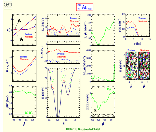
Gold 210 (Z=79, N=131)
