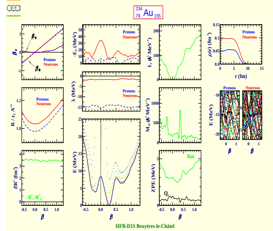
Gold 234 (Z=79, N=155)
