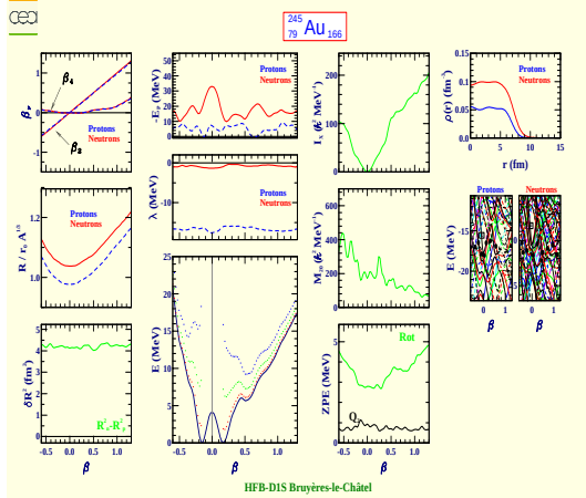
Gold 245 (Z=79, N=166)
