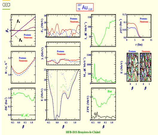
Gold 197 (Z=79, N=118)
