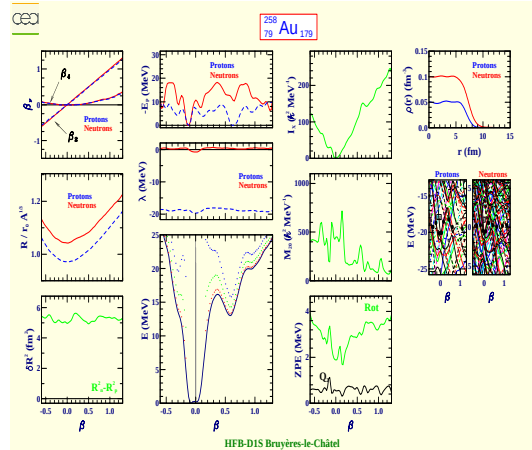
Or 258 (Z=79, N=179)
