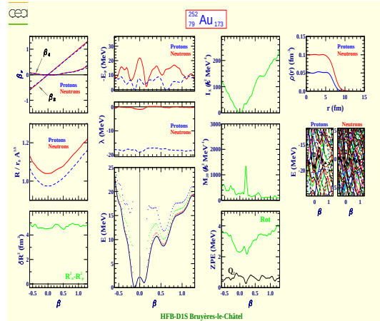
Or 252 (Z=79, N=173)
