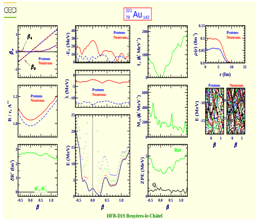
Or 221 (Z=79, N=142)
