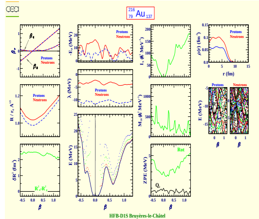
Or 216 (Z=79, N=137)
