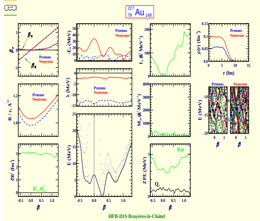
Or 227 (Z=79, N=148)
