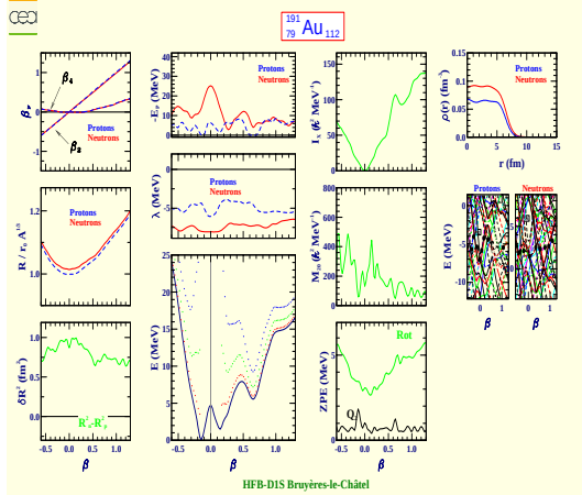
Or 191 (Z=79, N=112)
