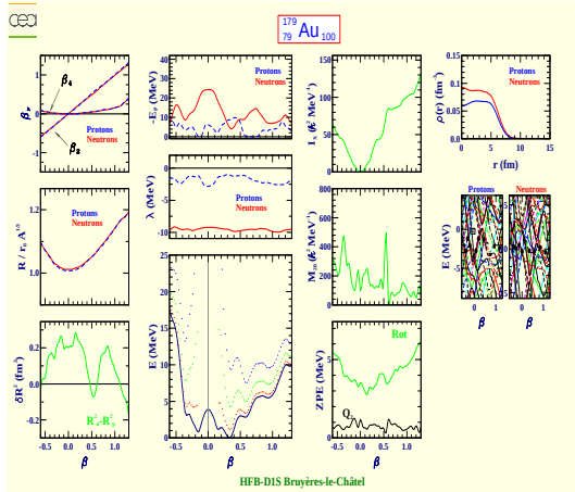
Or 179 (Z=79, N=100)
