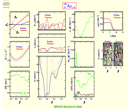
Or 198 (Z=79, N=119)
