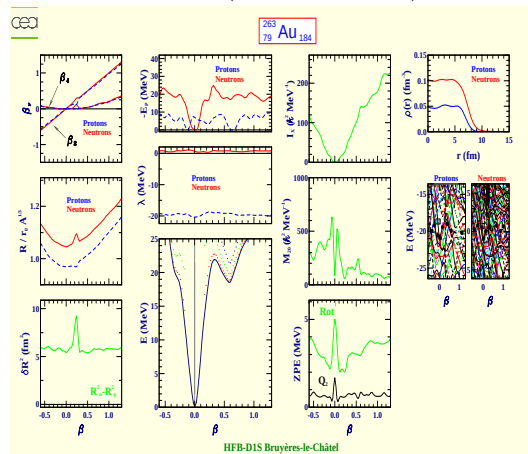
Or 263 (Z=79, N=184)
