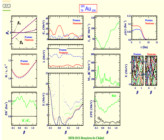
Or 185 (Z=79, N=106)
