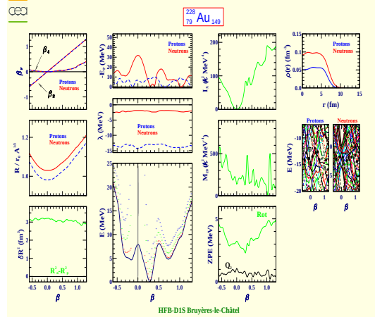
Or 228 (Z=79, N=149)
