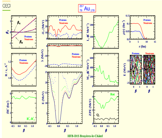
Or 257 (Z=79, N=178)
