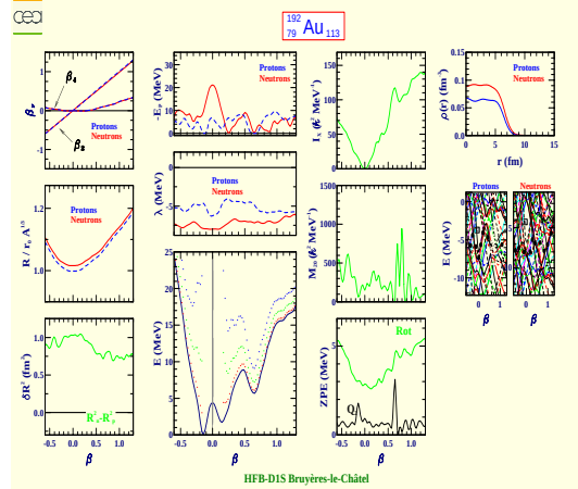
Or 192 (Z=79, N=113)
