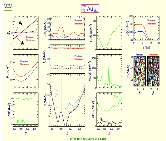
Or 240 (Z=79, N=161)
