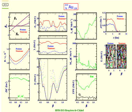
Or 215 (Z=79, N=136)
