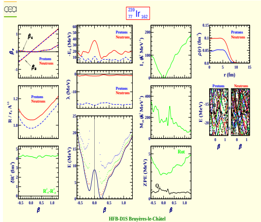
Iridium 239 (Z=77, N=162)
