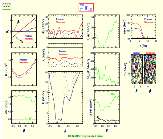
Iridium 197 (Z=77, N=120)
