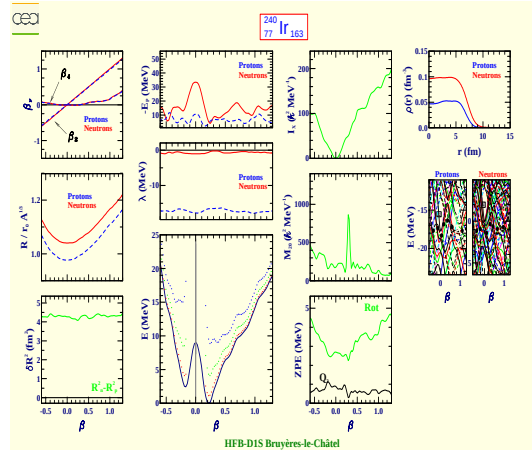
Iridium 240 (Z=77, N=163)
