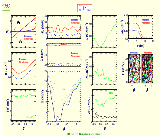
Iridium 251 (Z=77, N=174)
