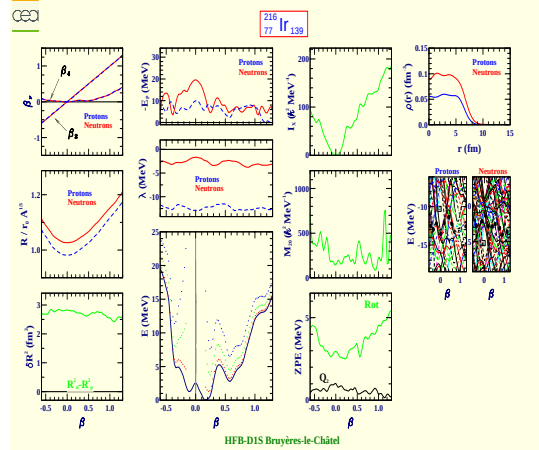
Iridium 216 (Z=77, N=139)
