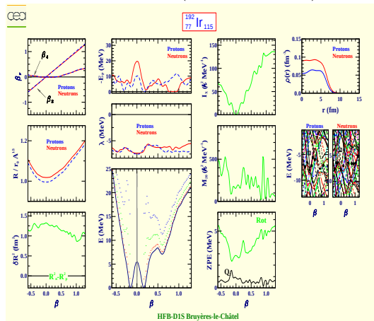
Iridium 192 (Z=77, N=115)
