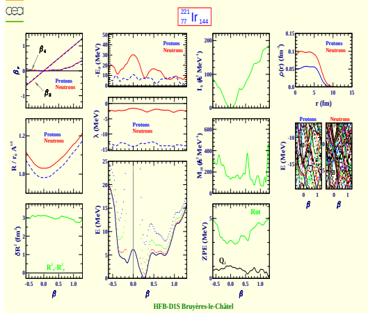
Iridium 221 (Z=77, N=144)
