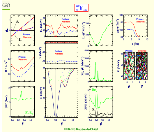
Iridium 260 (Z=77, N=183)
