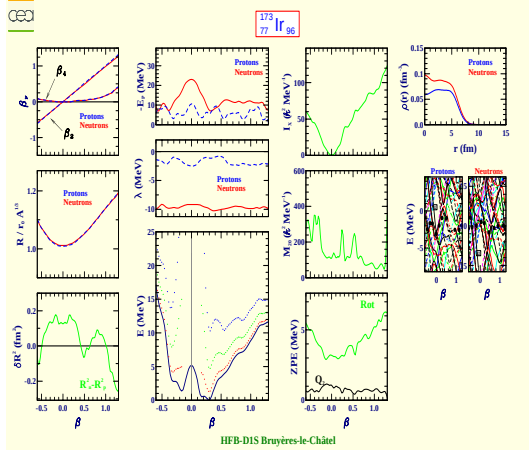
Iridium 173 (Z=77, N=96)
