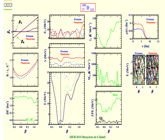
Iridium 198 (Z=77, N=121)
