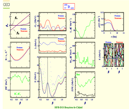
Iridium 180 (Z=77, N=103)
