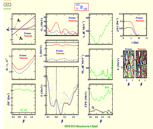
Iridium 222 (Z=77, N=145)
