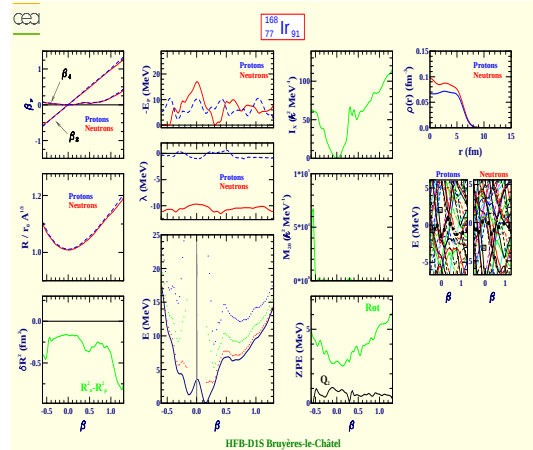
Iridium 168 (Z=77, N=91)
