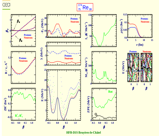
Rhénium 174 (Z=75, N=99)
