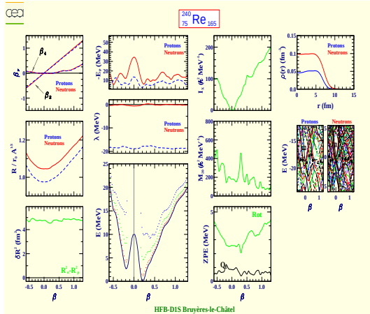
Rhénium 240 (Z=75, N=165)
