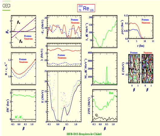
Rhénium 210 (Z=75, N=135)
