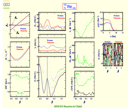
Rhénium 181 (Z=75, N=106)
