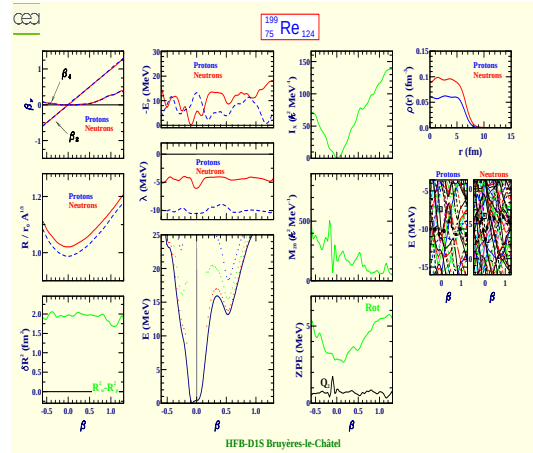
Rhénium 199 (Z=75, N=124)
