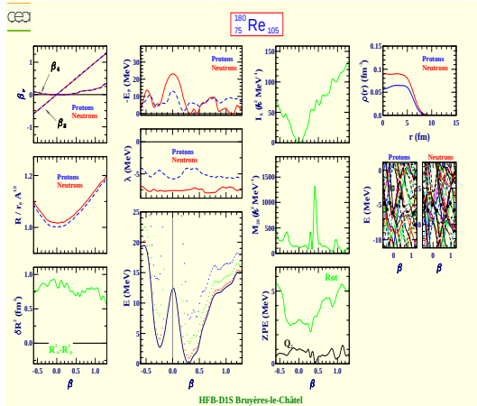
Rhénium 180 (Z=75, N=105)
