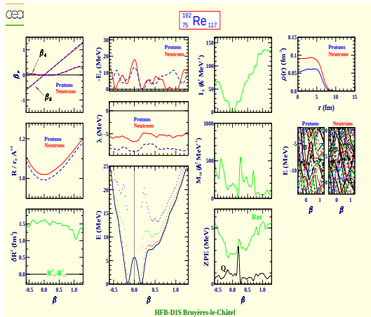
Rhénium 192 (Z=75, N=117)
