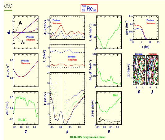
Rhénium 169 (Z=75, N=94)
