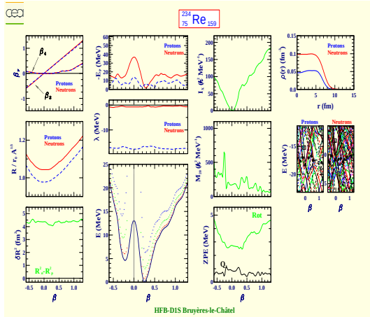
Rhénium 234 (Z=75, N=159)
