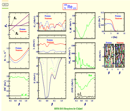
Rhénium 198 (Z=75, N=123)
