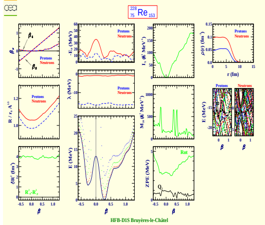
Rhénium 228 (Z=75, N=153)
