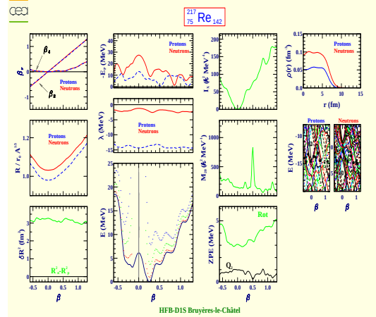
Rhénium 217 (Z=75, N=142)
