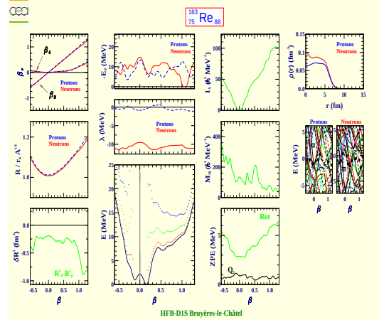
Rhénium 163 (Z=75, N=88)
