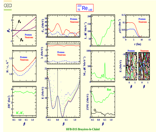
Rhénium 223 (Z=75, N=148)
