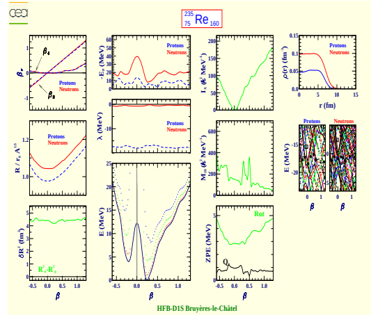
Rhénium 235 (Z=75, N=160)
