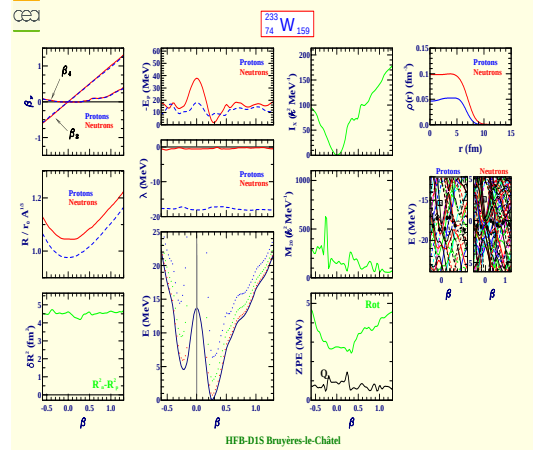
Tungstène 233 (Z=74, N=159)
