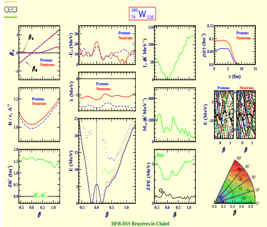
Tungstène 190 (Z=74, N=116)
