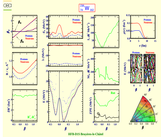
Tungstène 236 (Z=74, N=162)
