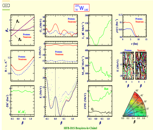
Tungstène 220 (Z=74, N=146)
