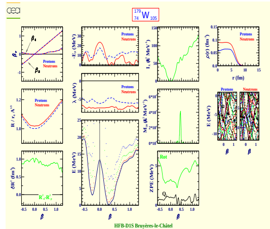
Tungstène 179 (Z=74, N=105)
