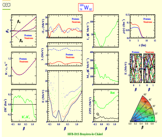
Tungstène 166 (Z=74, N=92)
