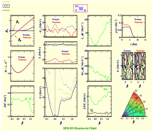
Tungstène 160 (Z=74, N=86)
