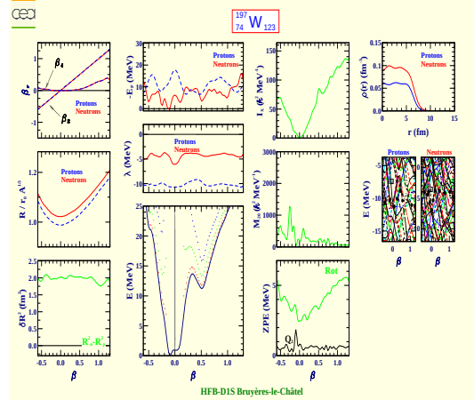
Tungstène 197 (Z=74, N=123)
