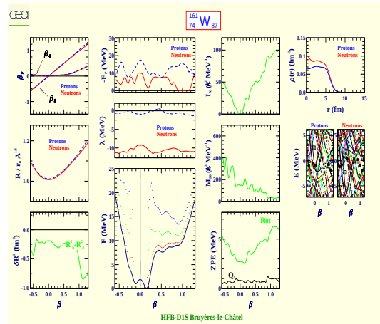
Tungstène 161 (Z=74, N=87)
