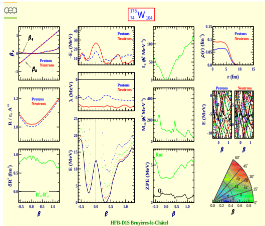
Tungstène 178 (Z=74, N=104)
