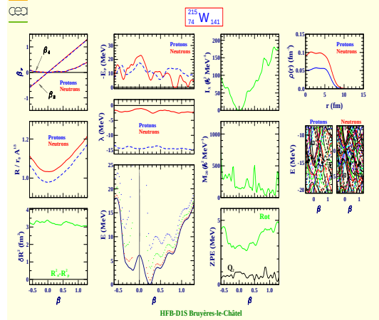
Tungstène 215 (Z=74, N=141)
