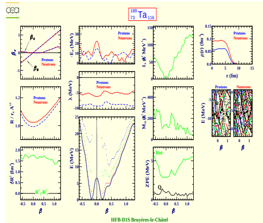
Tantale 189 (Z=73, N=116)
