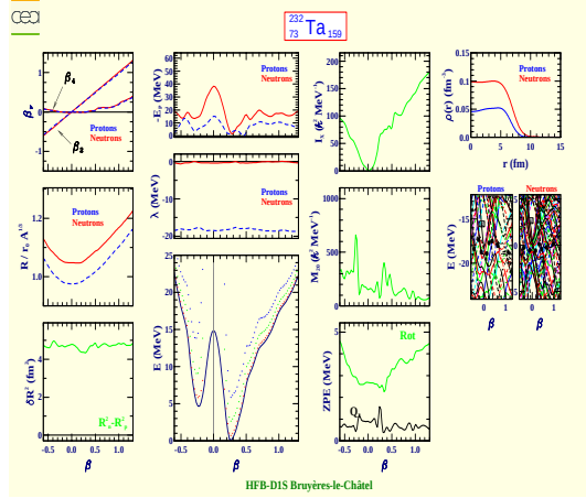
Tantale 232 (Z=73, N=159)
