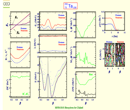
Tantale 231 (Z=73, N=158)
