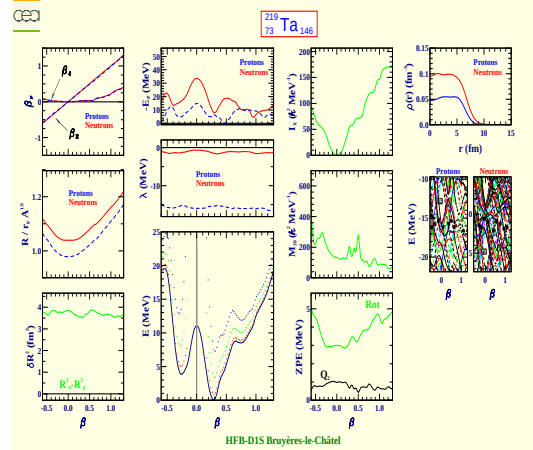
Tantale 219 (Z=73, N=146)
