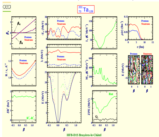
Tantale 201 (Z=73, N=128)
