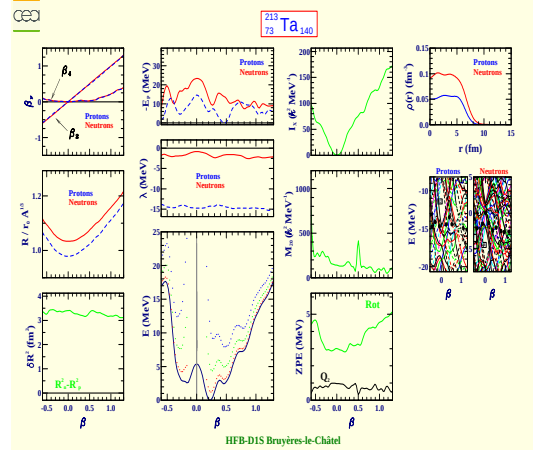
Tantale 213 (Z=73, N=140)
