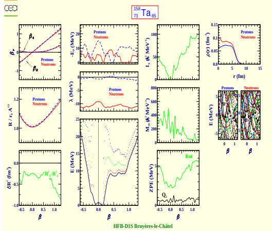
Tantale 158 (Z=73, N=85)
