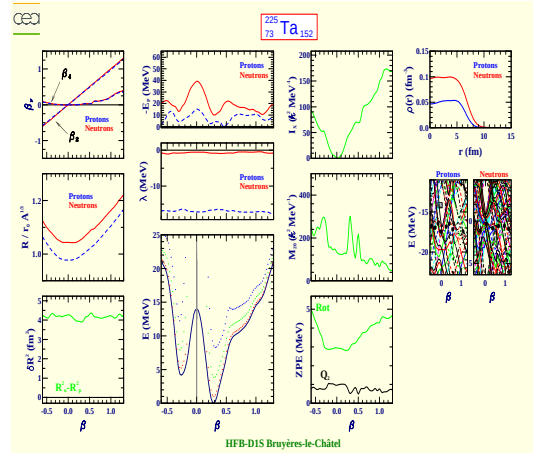
Tantale 225 (Z=73, N=152)
