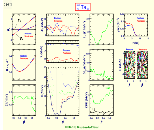
Tantale 159 (Z=73, N=86)
