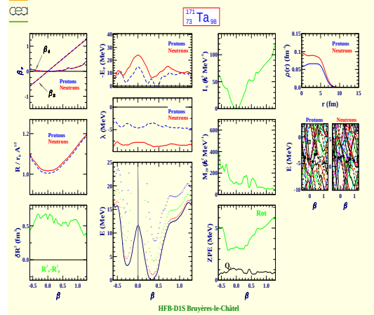
Tantale 171 (Z=73, N=98)
