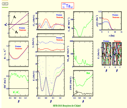
Tantale 170 (Z=73, N=97)
