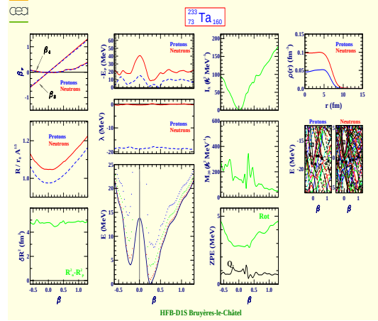
Tantale 233 (Z=73, N=160)
