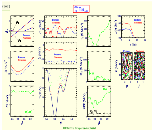
Tantale 200 (Z=73, N=127)
