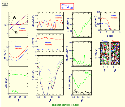
Tantale 206 (Z=73, N=133)
