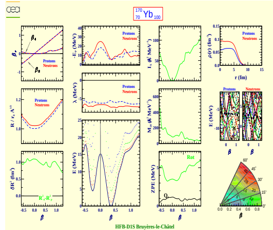
Yterbium 170 (Z=70, N=100)
