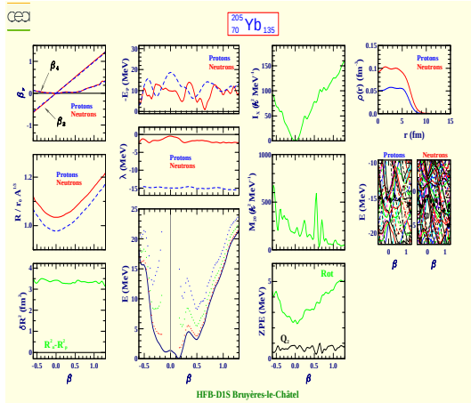
Yterbium 205 (Z=70, N=135)
