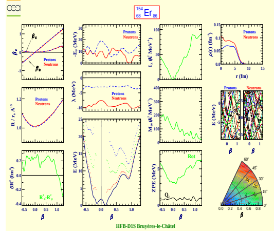
Erbium 154 (Z=68, N=86)
