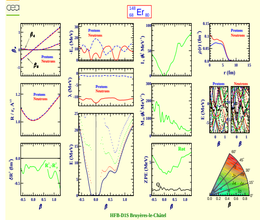
Erbium 148 (Z=68, N=80)
