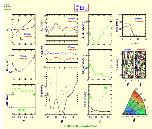
Erbium 160 (Z=68, N=92)
