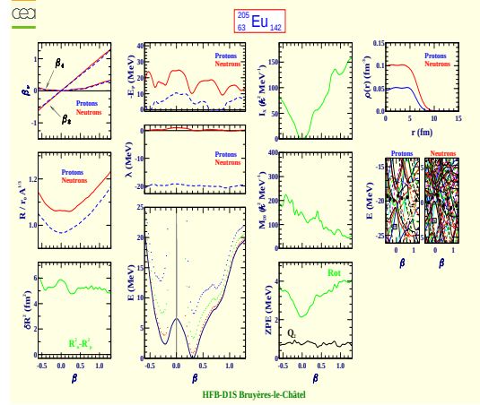
Europium 205 (Z=63, N=142)
