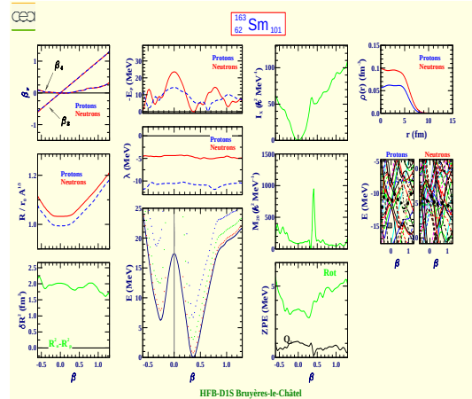
Samarium 163 (Z=62, N=101)
