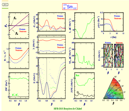
Samarium 174 (Z=62, N=112)
