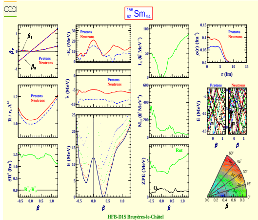
Samarium 156 (Z=62, N=94)
