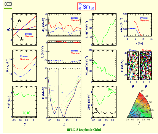
Samarium 204 (Z=62, N=142)
