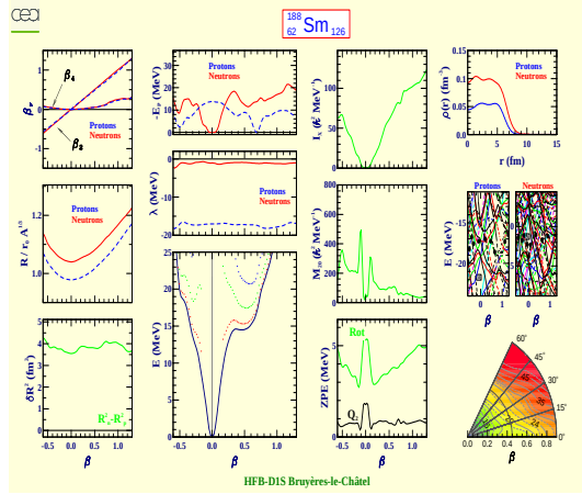
Samarium 188 (Z=62, N=126)
