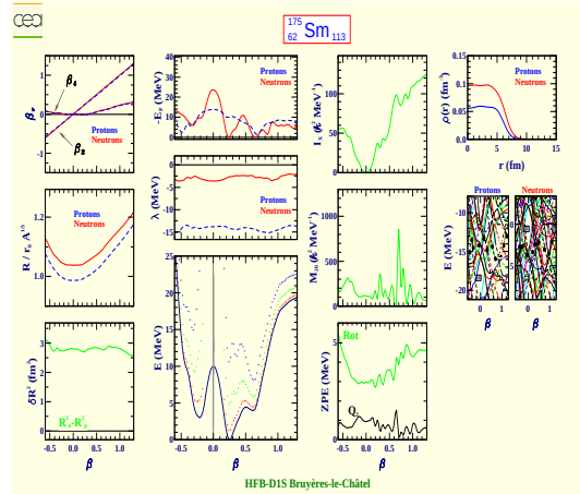
Samarium 175 (Z=62, N=113)
