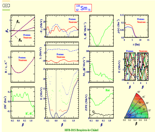
Samarium 138 (Z=62, N=76)
