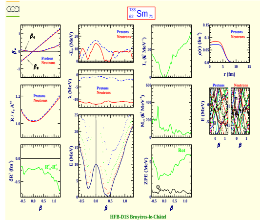
Samarium 133 (Z=62, N=71)
