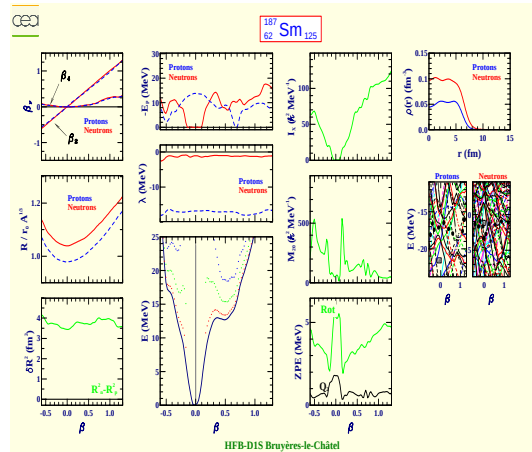
Samarium 187 (Z=62, N=125)
