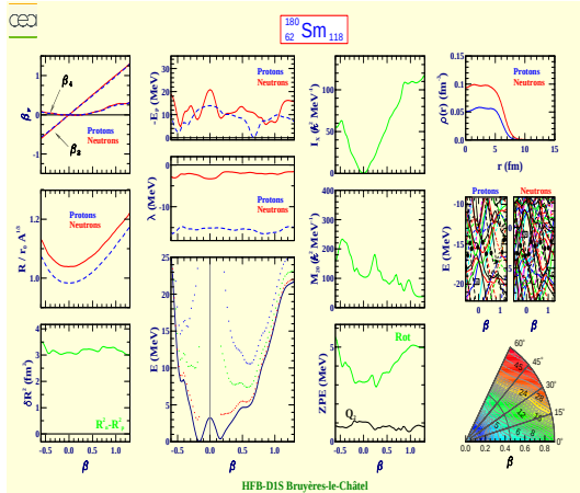
Samarium 180 (Z=62, N=118)
