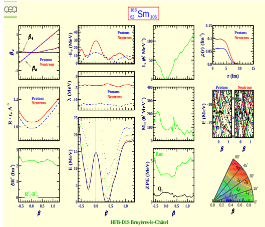
Samarium 168 (Z=62, N=106)
