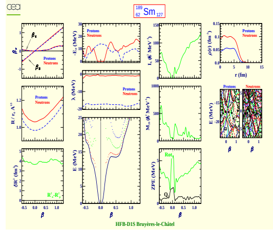
Samarium 189 (Z=62, N=127)
