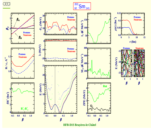
Samarium 203 (Z=62, N=141)
