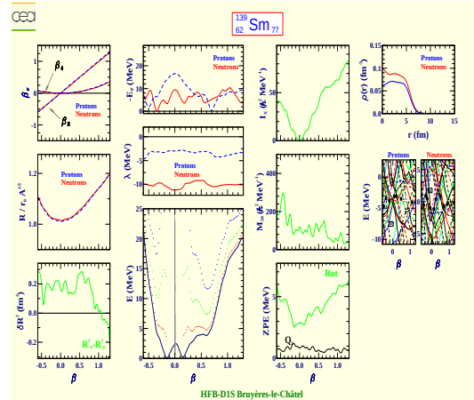
Samarium 139 (Z=62, N=77)
