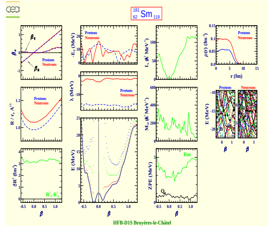
Samarium 181 (Z=62, N=119)
