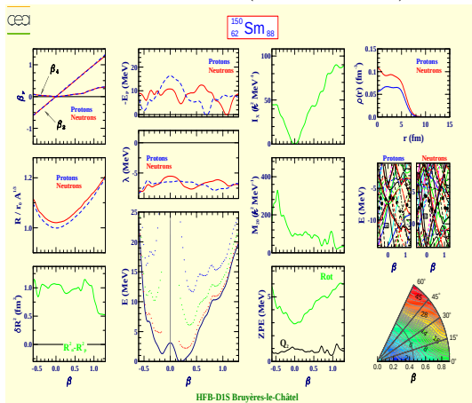
Samarium 150 (Z=62, N=88)
