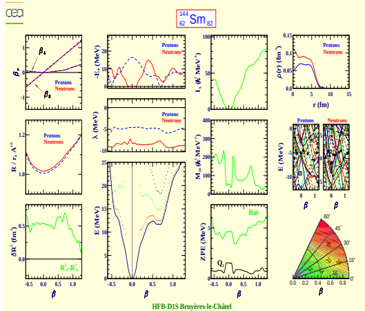
Samarium 144 (Z=62, N=82)
