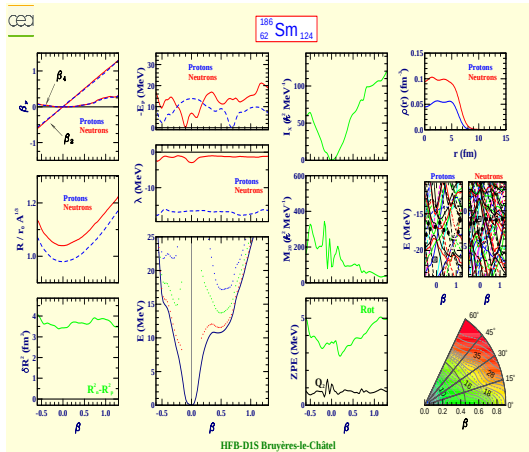
Samarium 186 (Z=62, N=124)
