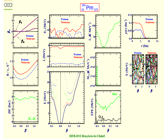
Prométhéum 184 (Z=61, N=123)
