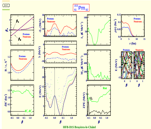
Prométhéum 153 (Z=61, N=92)
