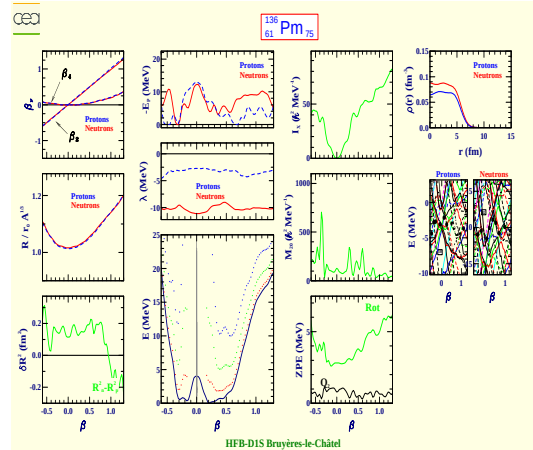
Prométhéum 136 (Z=61, N=75)
