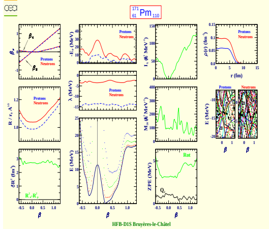
Prométhéum 171 (Z=61, N=110)
