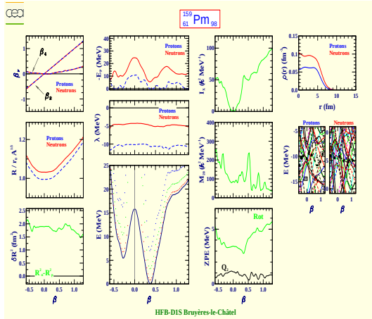
Prométhéum 159 (Z=61, N=98)
