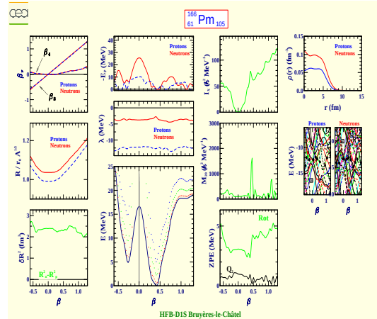
Prométhéum 166 (Z=61, N=105)
