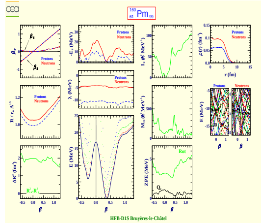
Prométhéum 160 (Z=61, N=99)
