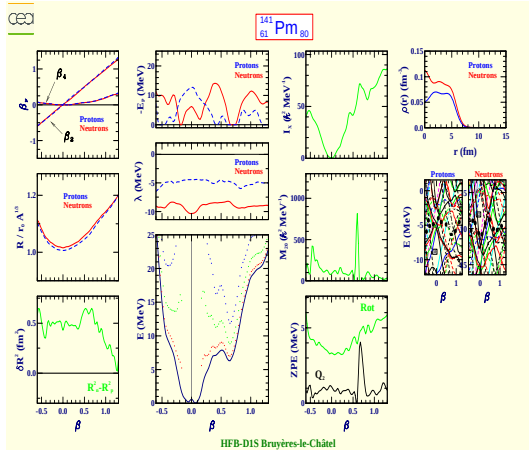
Prométhéum 141 (Z=61, N=80)
