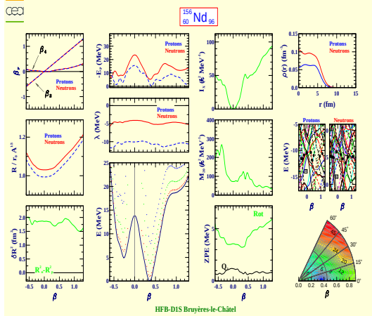
Néodyme 156 (Z=60, N=96)
