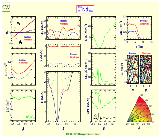
Néodyme 186 (Z=60, N=126)
