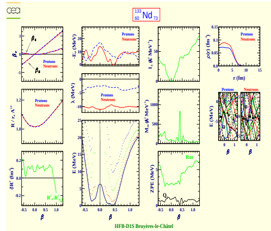
Néodyme 133 (Z=60, N=73)
