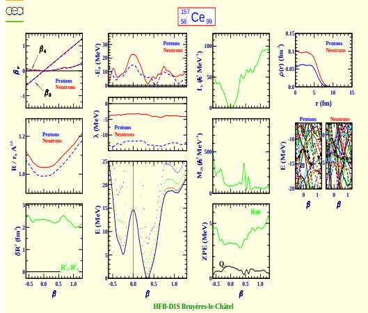
Cérium 157 (Z=58, N=99)
