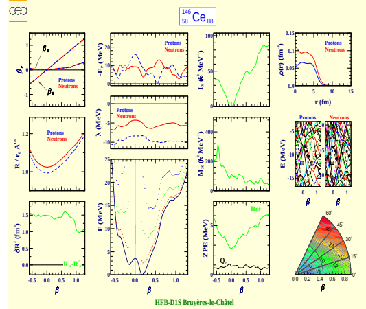
Cérium 146 (Z=58, N=88)
