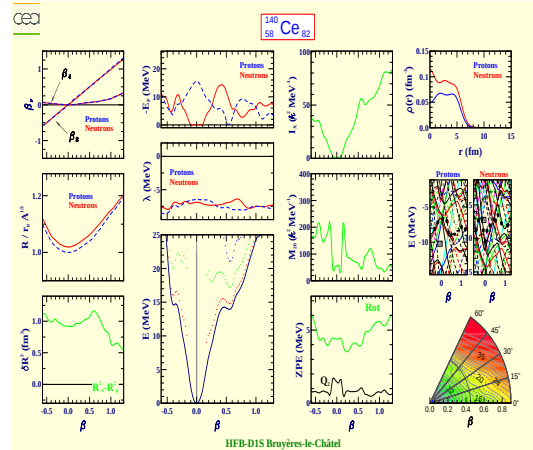
Cérium 140 (Z=58, N=82)
