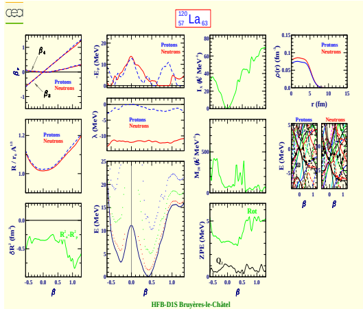
Lanthane 120 (Z=57, N=63)
