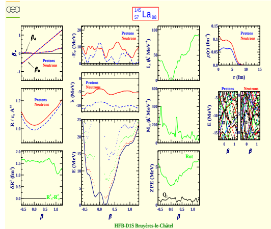
Lanthane 145 (Z=57, N=88)
