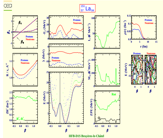
Lanthane 151 (Z=57, N=94)
