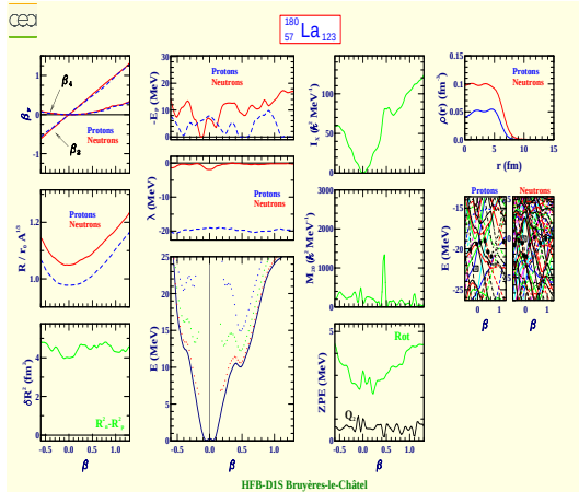
Lanthane 180 (Z=57, N=123)
