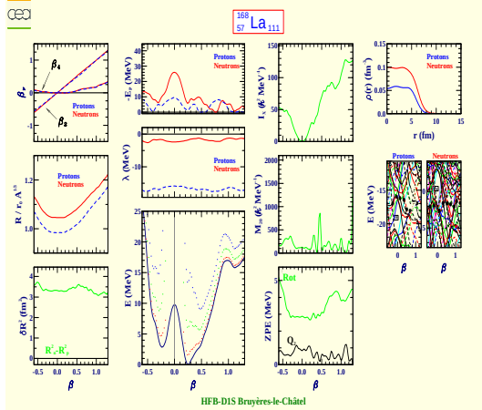
Lanthane 168 (Z=57, N=111)
