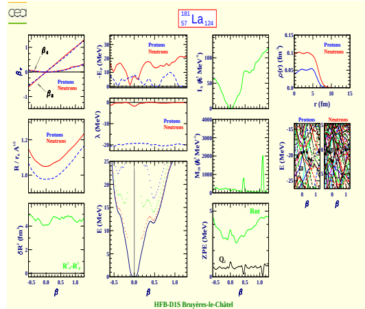
Lanthane 181 (Z=57, N=124)
