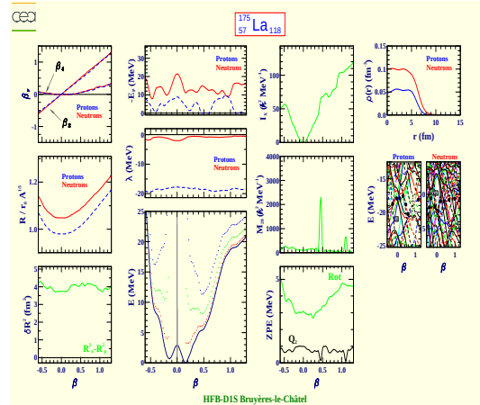
Lanthane 175 (Z=57, N=118)
