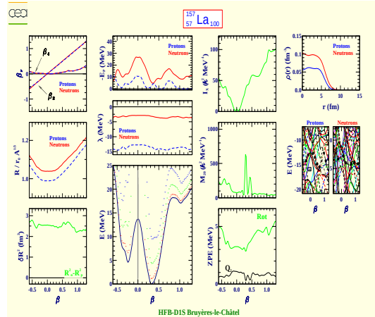
Lanthane 157 (Z=57, N=100)
