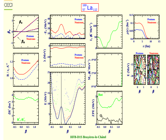
Lanthane 169 (Z=57, N=112)
