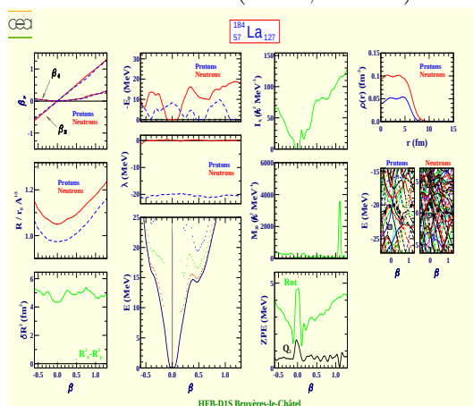
Lanthane 184 (Z=57, N=127)
