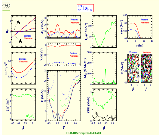
Lanthane 174 (Z=57, N=117)
