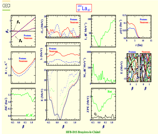
Lanthane 144 (Z=57, N=87)
