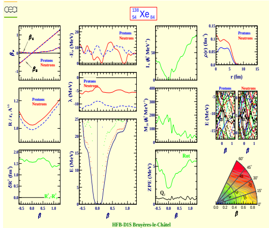
Xénon 138 (Z=54, N=84)
