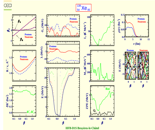
Xénon 139 (Z=54, N=85)
