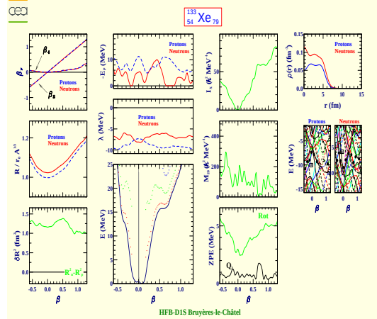
Xénon 133 (Z=54, N=79)
