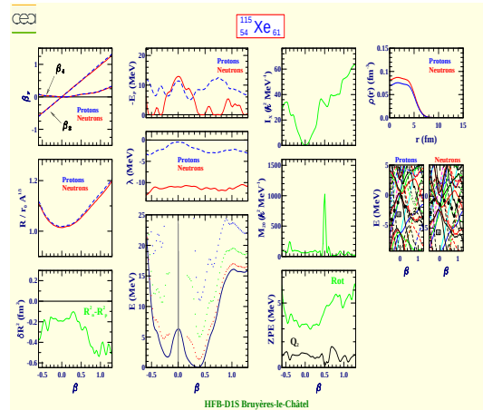
Xénon 115 (Z=54, N=61)
