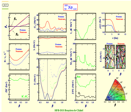
Xénon 168 (Z=54, N=114)
