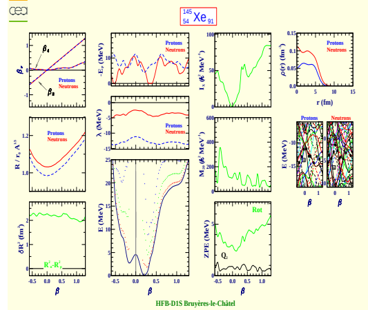
Xénon 145 (Z=54, N=91)
