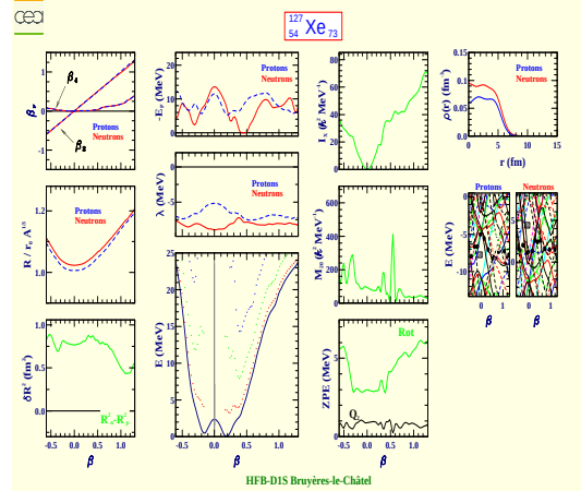
Xénon 127 (Z=54, N=73)
