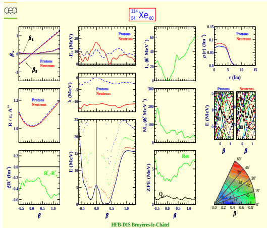
Xénon 114 (Z=54, N=60)
