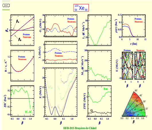
Xénon 120 (Z=54, N=66)
