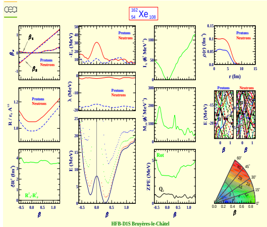
Xénon 162 (Z=54, N=108)
