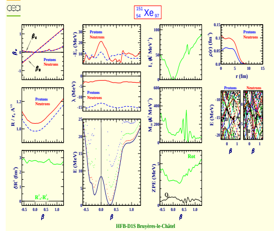
Xénon 151 (Z=54, N=97)
