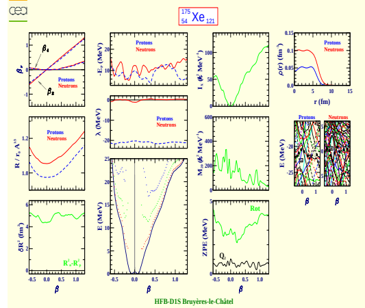
Xénon 175 (Z=54, N=121)
