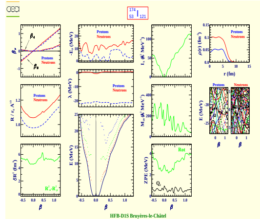
Iode 174 (Z=53, N=121)
