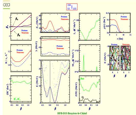
Iode 156 (Z=53, N=103)
