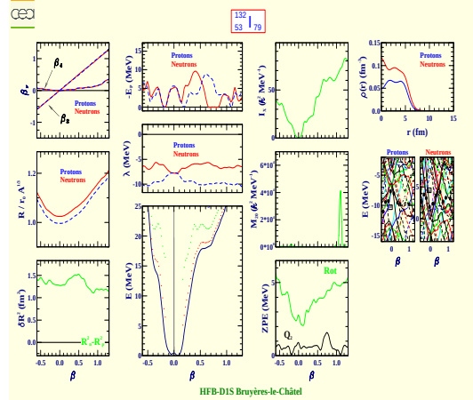
Iode 132 (Z=53, N=79)
