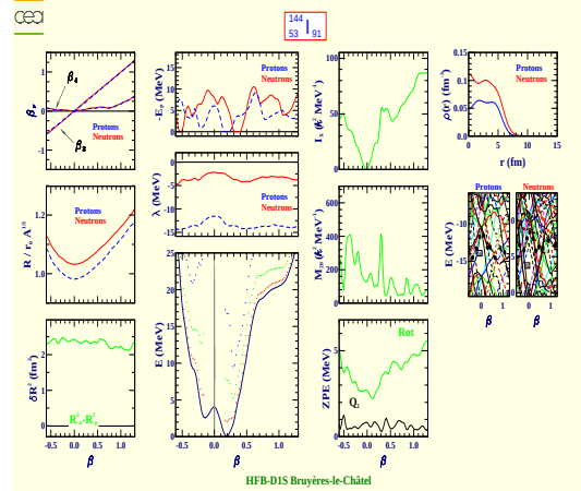
Iode 144 (Z=53, N=91)
