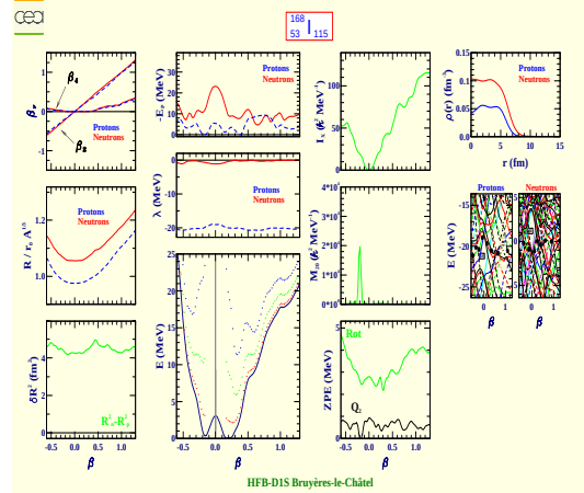
Iode 168 (Z=53, N=115)
