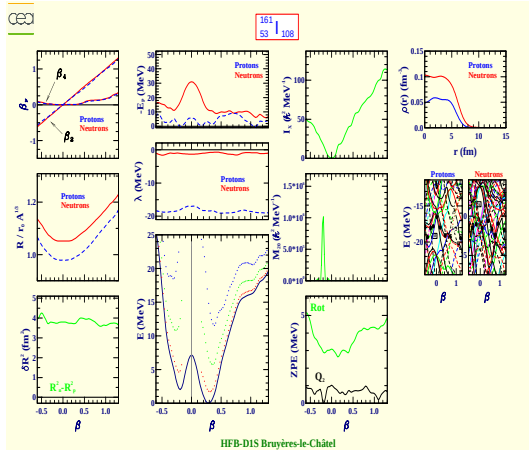
Iode 161 (Z=53, N=108)
