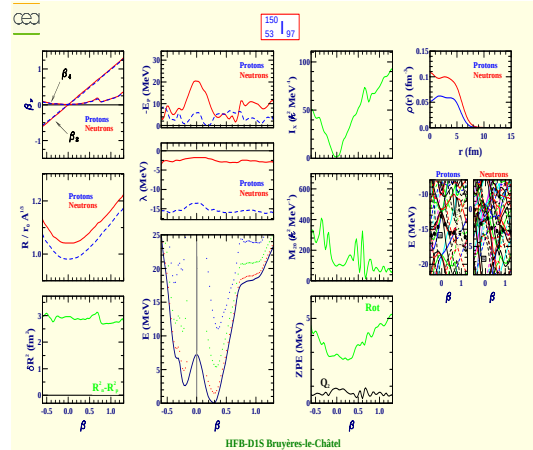
Iode 150 (Z=53, N=97)
