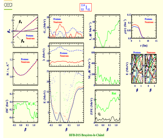
Iode 114 (Z=53, N=61)
