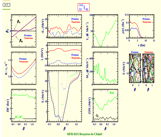
Iode 143 (Z=53, N=90)
