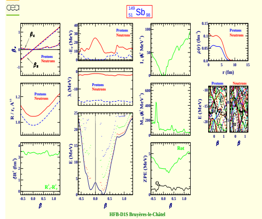
Antimoine 149 (Z=51, N=98)
