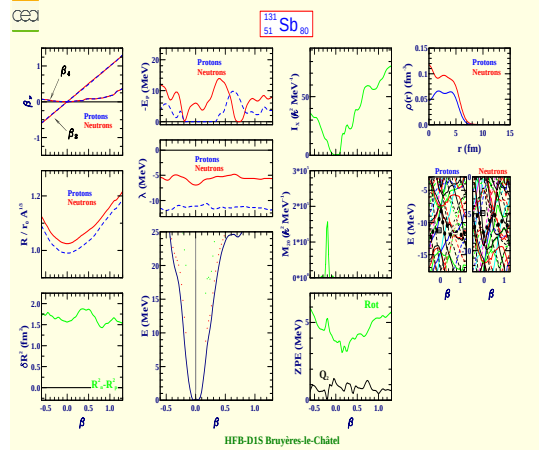
Antimoine 131 (Z=51, N=80)
