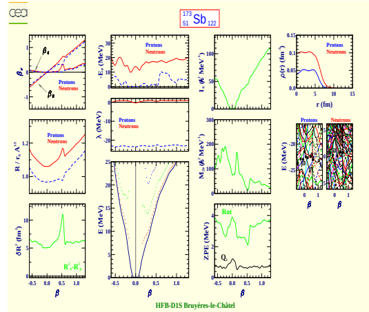
Antimoine 173 (Z=51, N=122)
