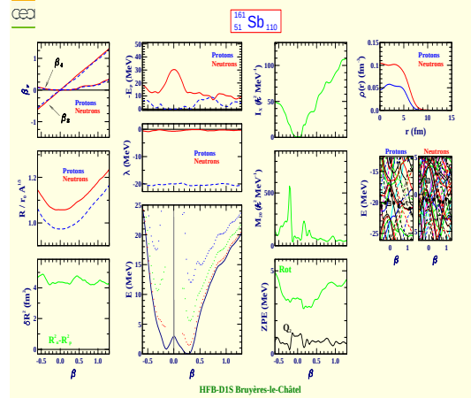
Antimoine 161 (Z=51, N=110)
