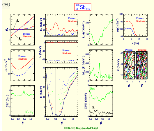
Antimoine 166 (Z=51, N=115)
