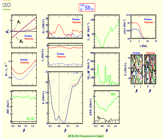
Antimoine 148 (Z=51, N=97)
