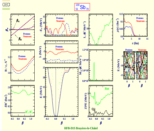
Antimoine 130 (Z=51, N=79)
