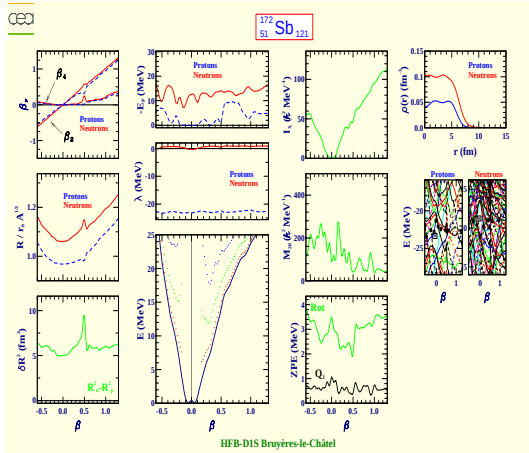
Antimoine 172 (Z=51, N=121)
