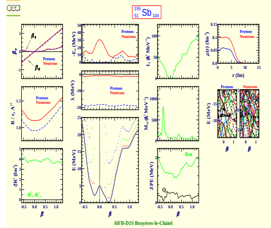
Antimoine 155 (Z=51, N=104)
