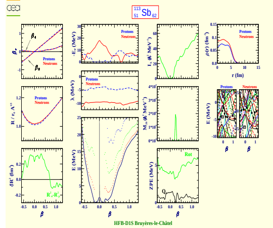
Antimoine 113 (Z=51, N=62)
