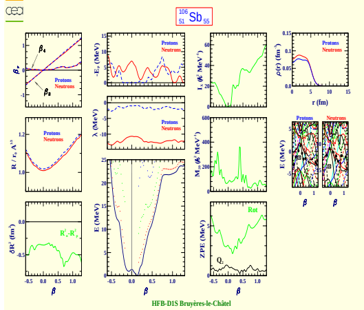
Antimoine 106 (Z=51, N=55)
