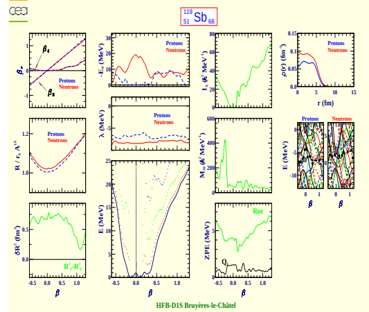
Antimoine 119 (Z=51, N=68)
