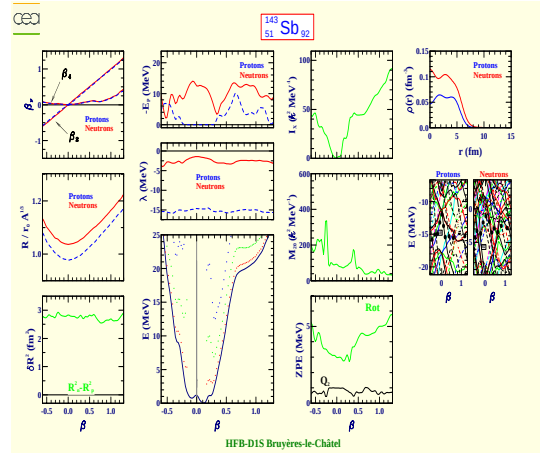
Antimoine 143 (Z=51, N=92)
