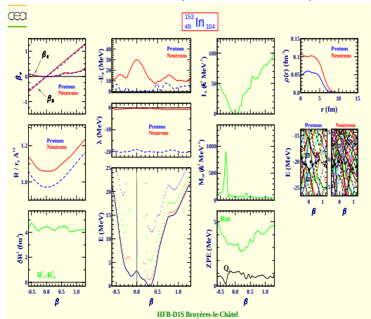
Indium 153 (Z=49, N=104)
