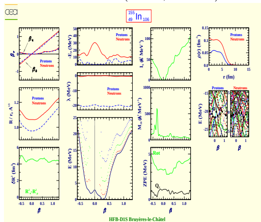
Indium 155 (Z=49, N=106)
