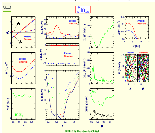
Indium 156 (Z=49, N=107)
