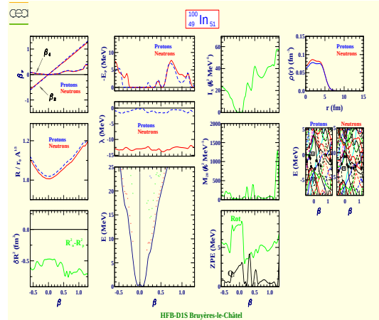
Indium 100 (Z=49, N=51)
