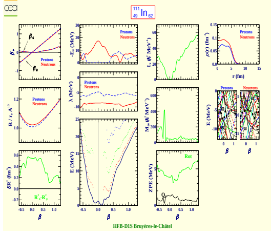
Indium 111 (Z=49, N=62)
