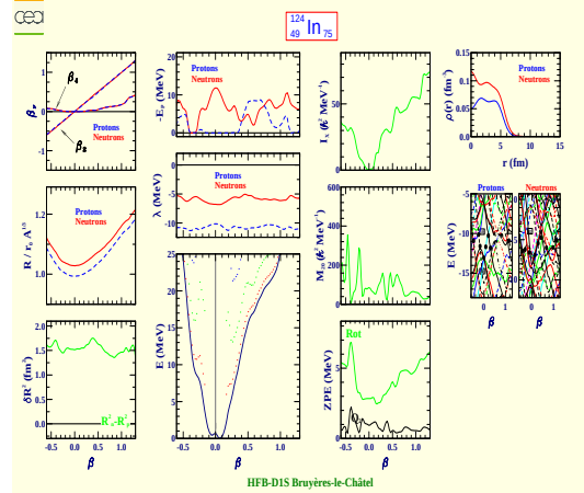
Indium 124 (Z=49, N=75)
