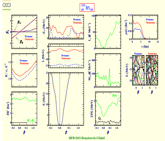
Indium 135 (Z=49, N=86)
