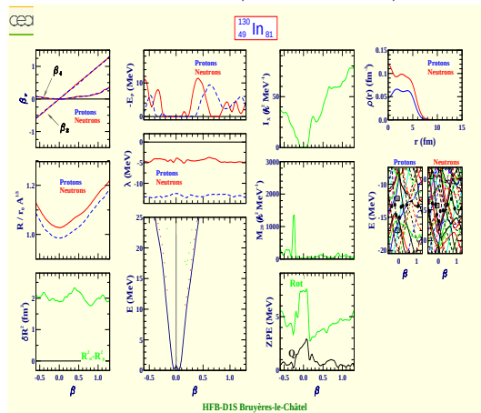
Indium 130 (Z=49, N=81)
