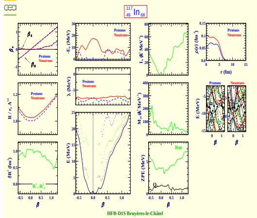
Indium 117 (Z=49, N=68)
