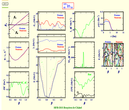
Indium 105 (Z=49, N=56)
