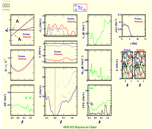
Technétium 87 (Z=43, N=44)
