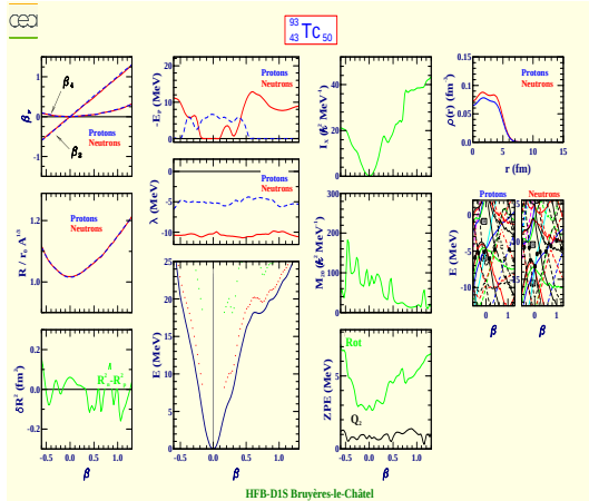
Technétium 93 (Z=43, N=50)
