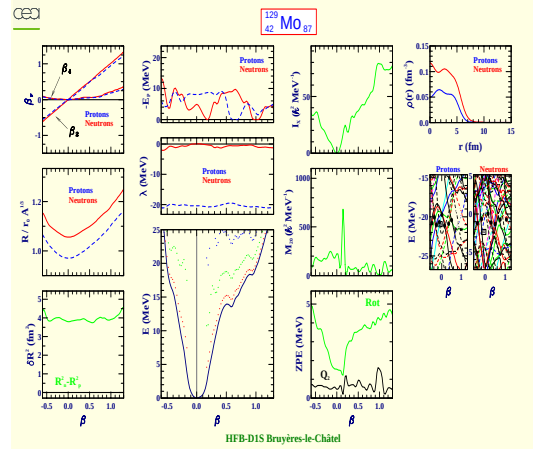
Molybdenum 129 (Z=42, N=87)
