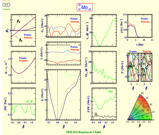
Molybdenum 90 (Z=42, N=48)
