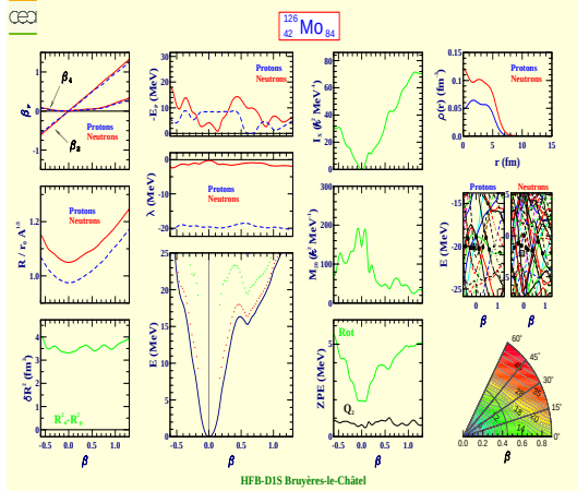
Molybdenum 126 (Z=42, N=84)
