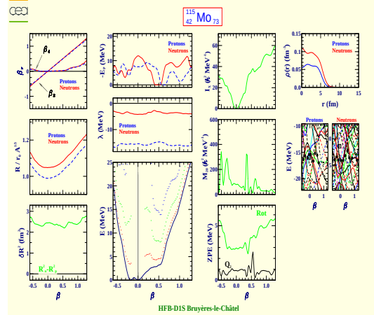
Molybdenum 115 (Z=42, N=73)
