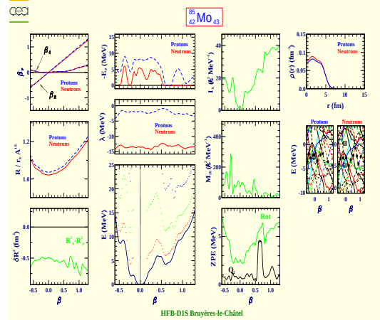
Molybdenum 85 (Z=42, N=43)
