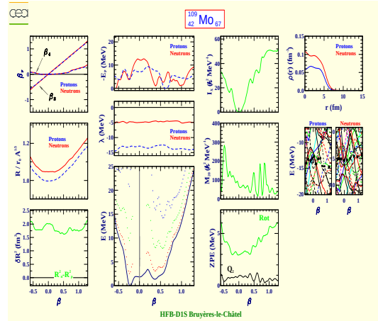
Molybdenum 109 (Z=42, N=67)
