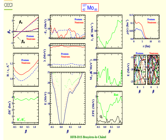
Molybdenum 127 (Z=42, N=85)
