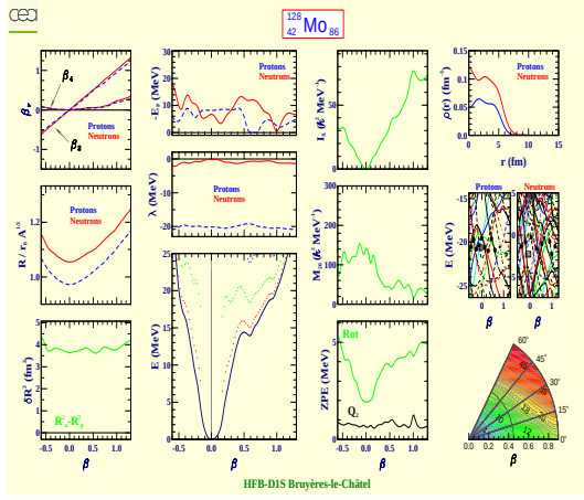
Molybdenum 128 (Z=42, N=86)
