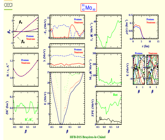
Molybdenum 91 (Z=42, N=49)
