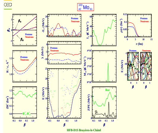
Molybdène 103 (Z=42, N=61)
