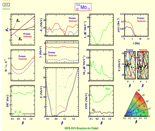
Molybdène 114 (Z=42, N=72)
