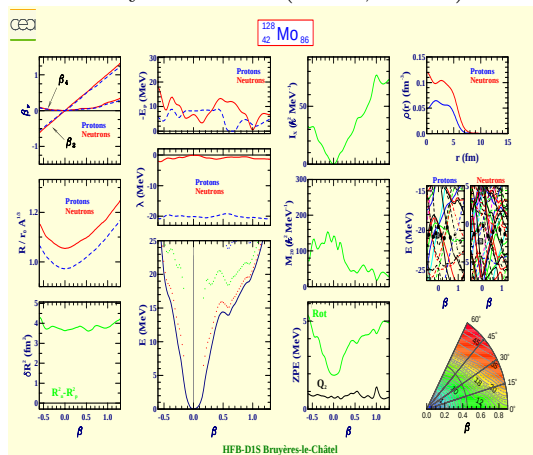
Molybdène 128 (Z=42, N=86)
