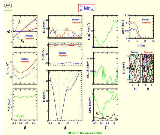
Molybdène 127 (Z=42, N=85)
