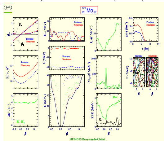
Molybdène 129 (Z=42, N=87)
