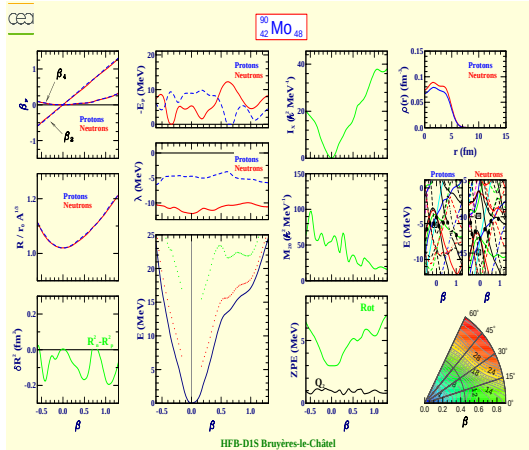
Molybdène 90 (Z=42, N=48)
