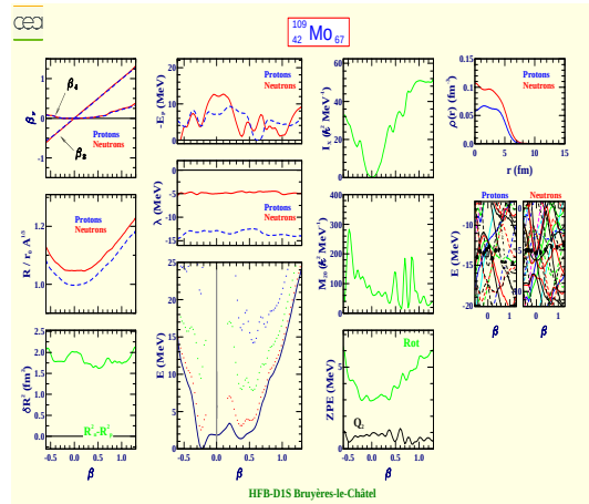
Molybdène 109 (Z=42, N=67)
