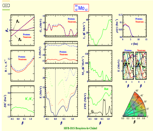
Molybdène 84 (Z=42, N=42)
