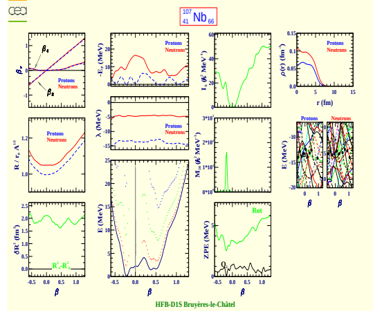
Niobium 107 (Z=41, N=66)
