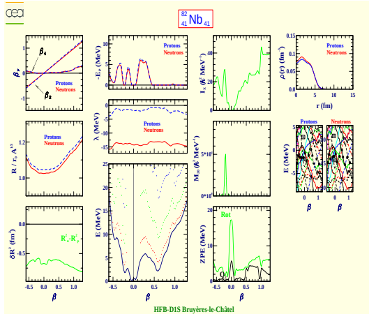
Niobium 82 (Z=41, N=41)
