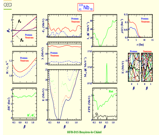
Niobium 119 (Z=41, N=78)
