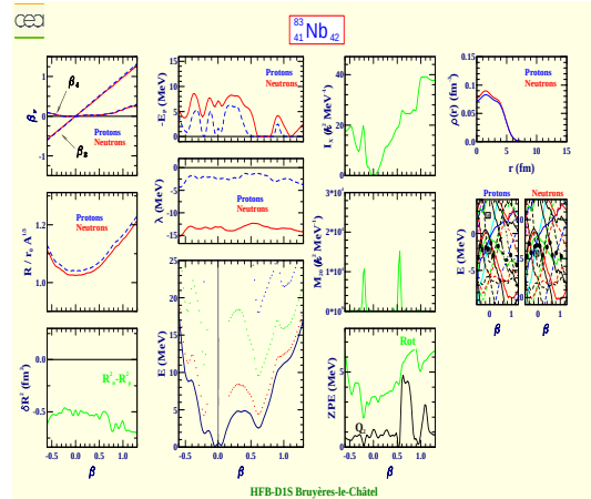
Niobium 83 (Z=41, N=42)
