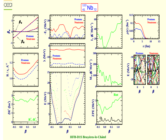
Niobium 113 (Z=41, N=72)
