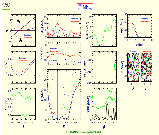
Niobium 100 (Z=41, N=59)
