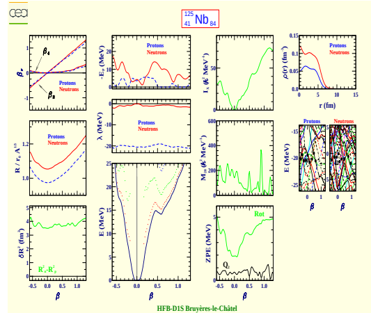
Niobium 125 (Z=41, N=84)
