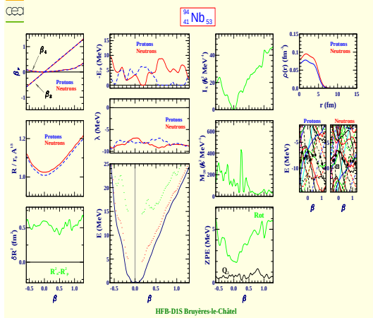
Niobium 94 (Z=41, N=53)
