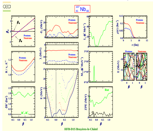
Niobium 107 (Z=41, N=66)
