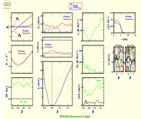
Niobium 95 (Z=41, N=54)
