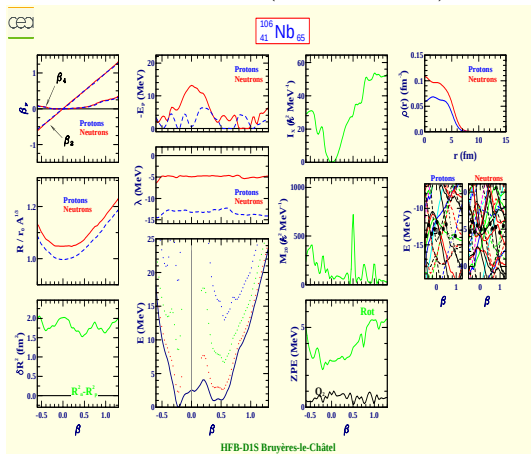
Niobium 106 (Z=41, N=65)
