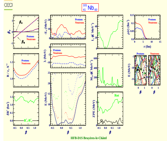
Niobium 101 (Z=41, N=60)
