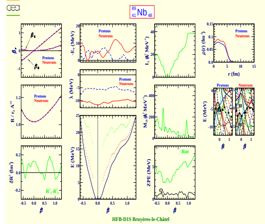
Niobium 89 (Z=41, N=48)
