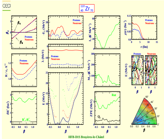
Zirconium 110 (Z=40, N=70)
