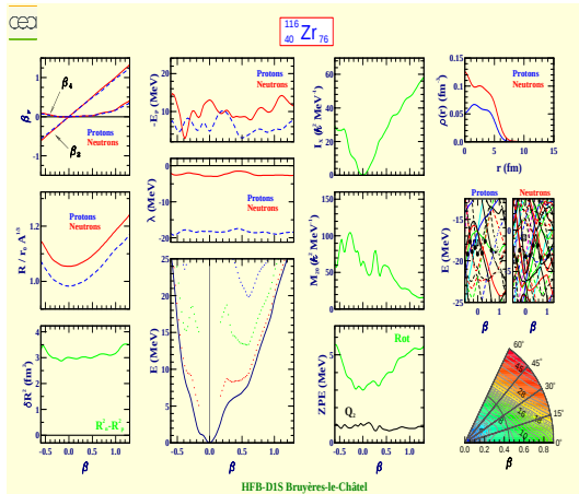
Zirconium 116 (Z=40, N=76)
