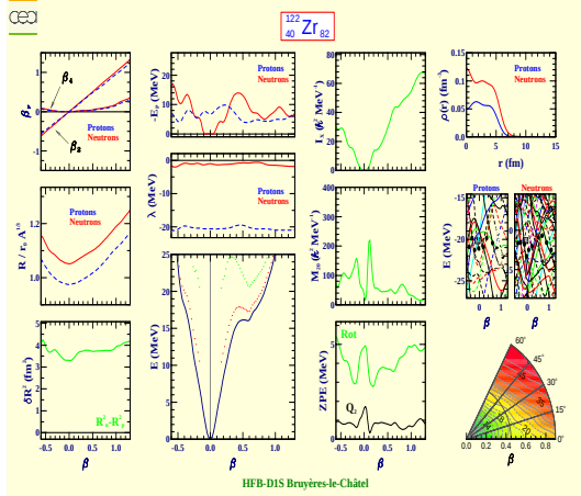
Zirconium 122 (Z=40, N=82)
