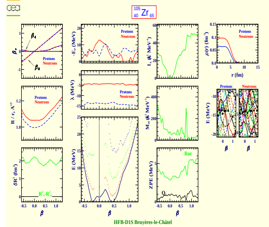
Zirconium 105 (Z=40, N=65)
