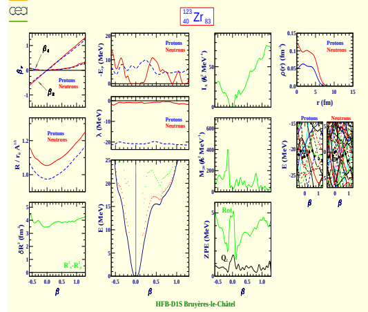
Zirconium 123 (Z=40, N=83)
