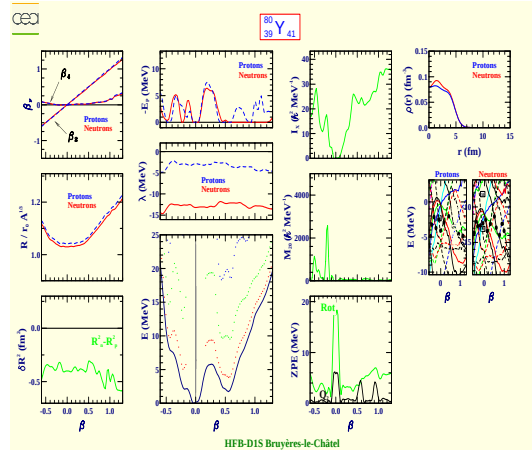
Yttrium 80 (Z=39, N=41)
