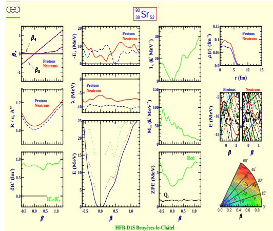
Strontium 90 (Z=38, N=52)
