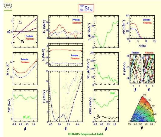
Strontium 102 (Z=38, N=64)
