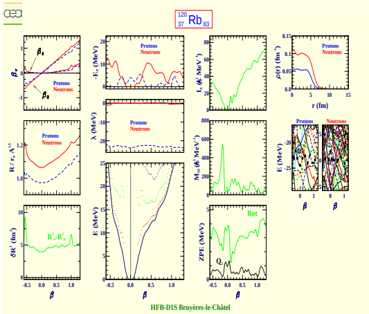
Rubidium 120 (Z=37, N=83)
