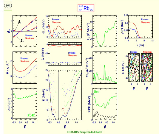
Rubidium 112 (Z=37, N=75)
