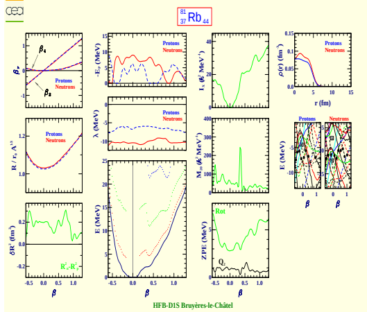
Rubidium 81 (Z=37, N=44)
