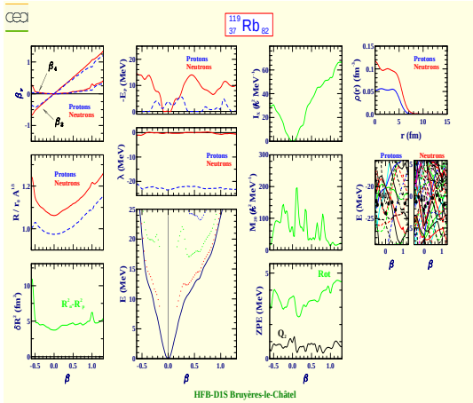
Rubidium 119 (Z=37, N=82)
