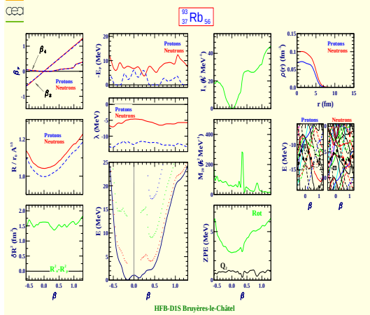
Rubidium 93 (Z=37, N=56)
