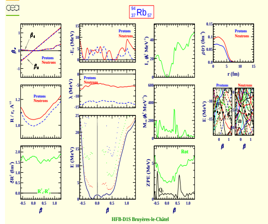
Rubidium 94 (Z=37, N=57)
