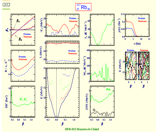
Rubidium 117 (Z=37, N=80)
