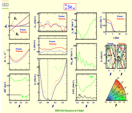
Sélénium 80 (Z=34, N=46)
