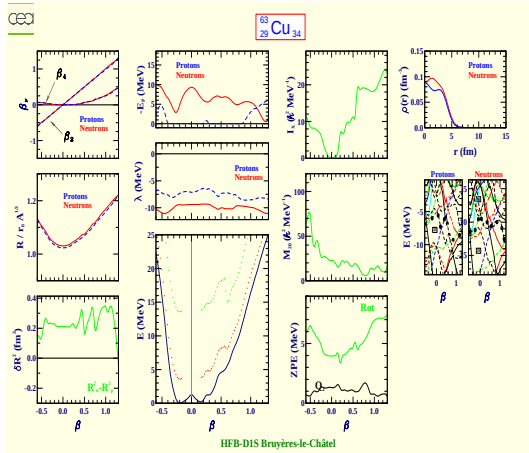
Cuivre 63 (Z=29, N=34)
