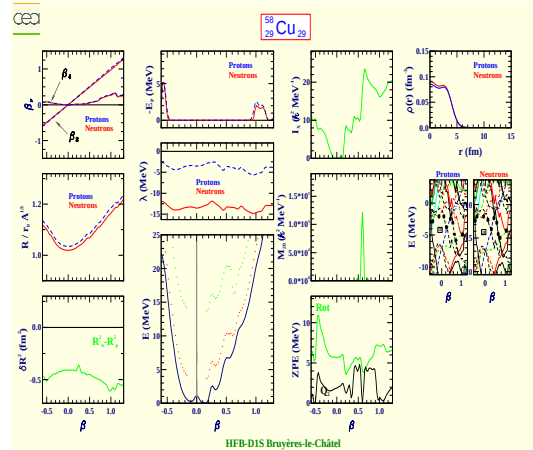
Cuivre 58 (Z=29, N=29)
