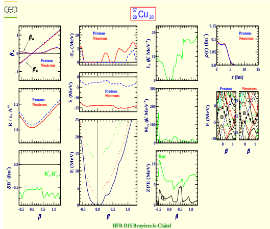
Cuivre 57 (Z=29, N=28)
