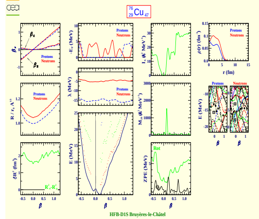
Cuivre 76 (Z=29, N=47)
