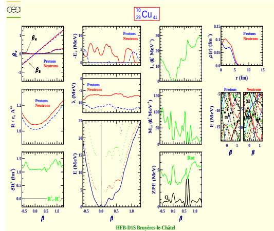
Cuivre 70 (Z=29, N=41)
