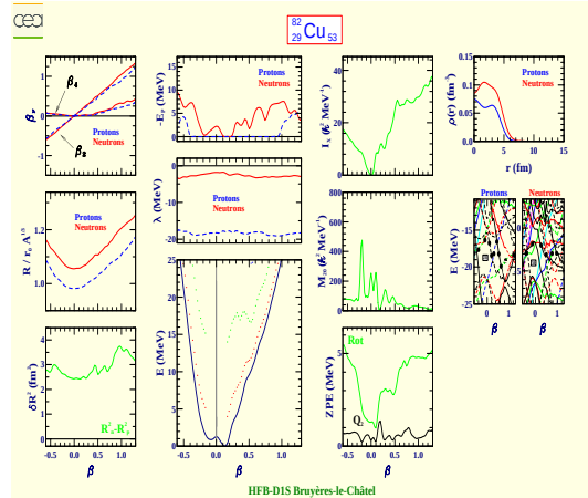
Cuivre 82 (Z=29, N=53)
