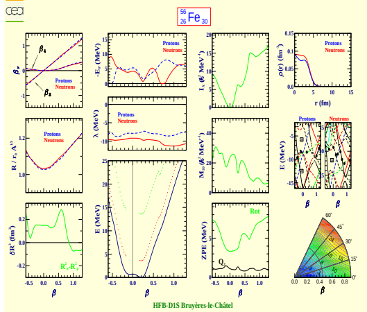
Iron 56 (Z=26, N=30)
