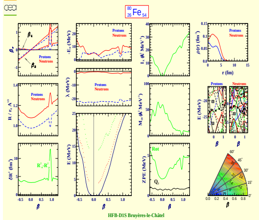
Iron 80 (Z=26, N=54)
