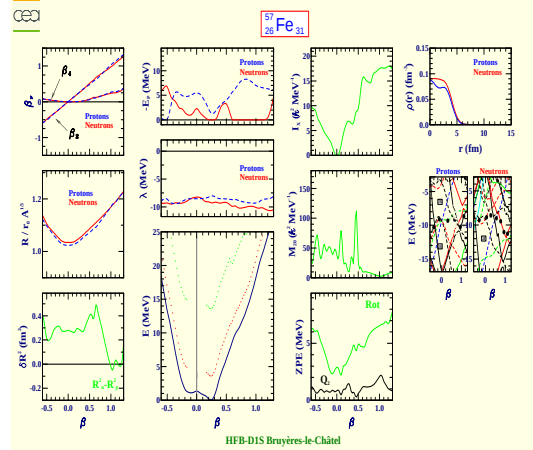
Iron 57 (Z=26, N=31)
