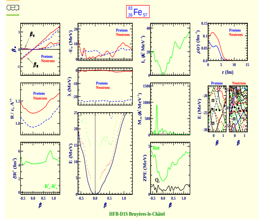
Iron 83 (Z=26, N=57)
