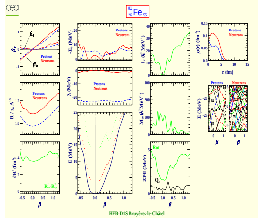
Iron 81 (Z=26, N=55)
