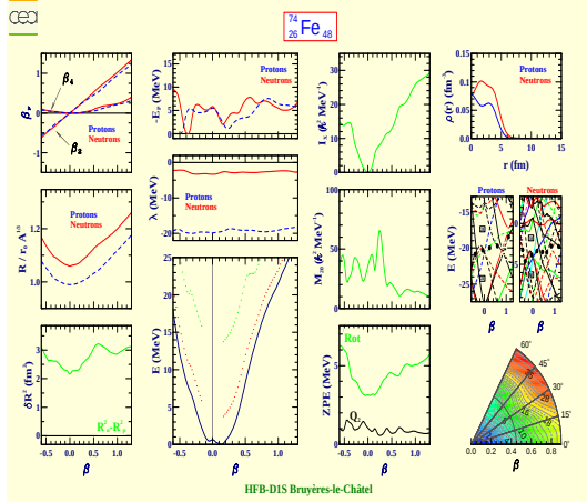
Iron 74 (Z=26, N=48)
