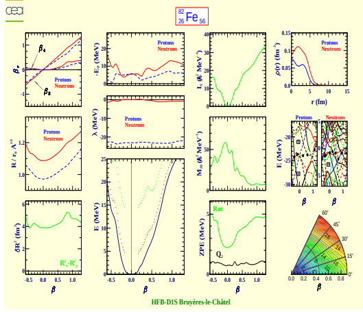
Iron 82 (Z=26, N=56)
