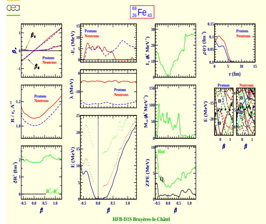
Iron 69 (Z=26, N=43)
