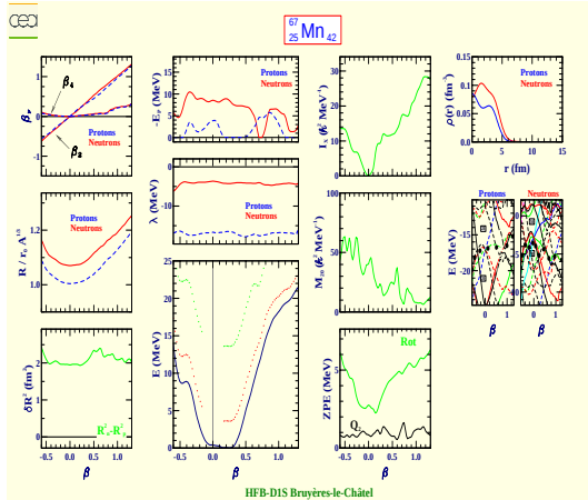
Manganèse 67 (Z=25, N=42)
