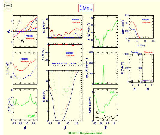
Manganèse 80 (Z=25, N=55)
