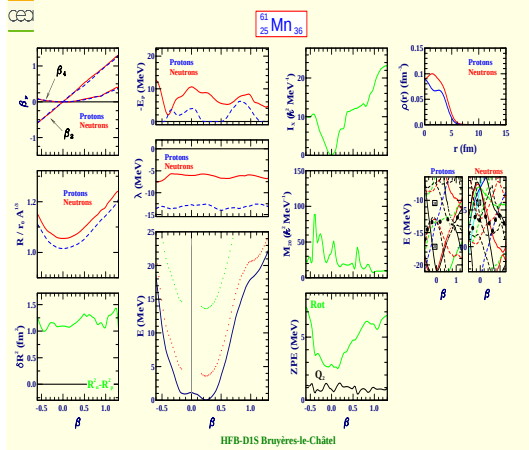
Manganèse 61 (Z=25, N=36)
