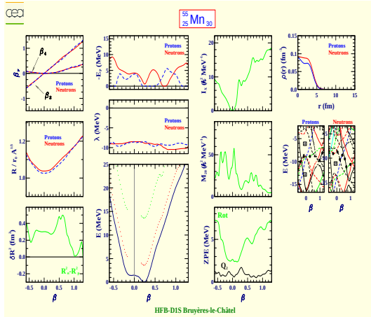
Manganèse 55 (Z=25, N=30)
