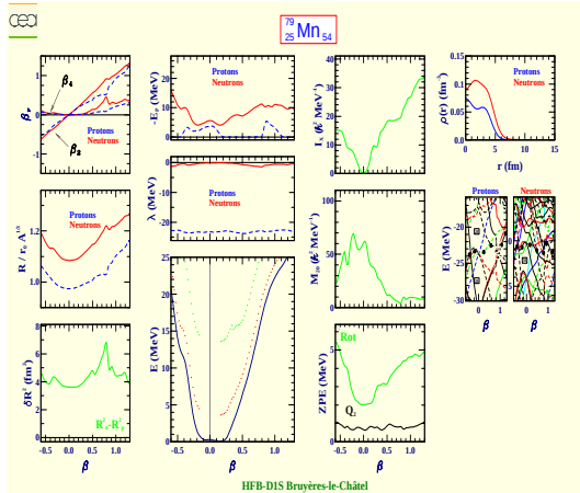
Manganèse 79 (Z=25, N=54)
