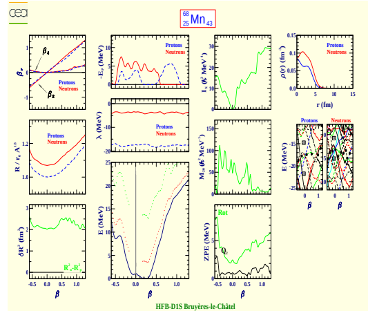
Manganèse 68 (Z=25, N=43)
