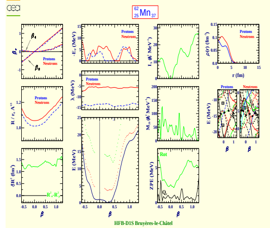
Manganèse 62 (Z=25, N=37)
