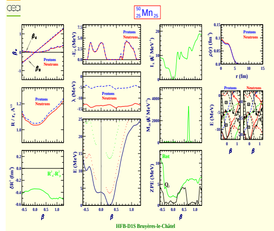
Manganèse 50 (Z=25, N=25)
