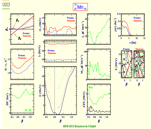
Manganèse 73 (Z=25, N=48)
