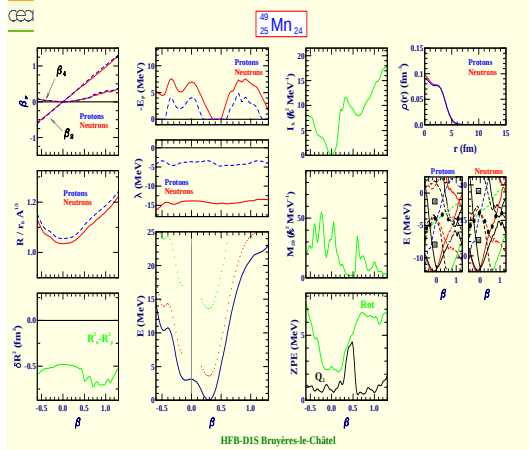
Manganèse 49 (Z=25, N=24)
