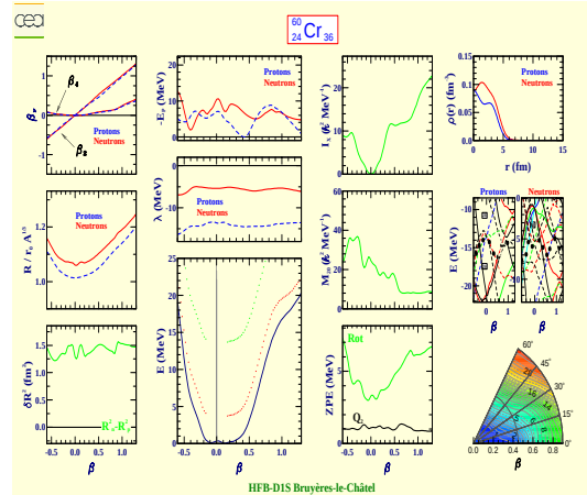
Chrome 60 (Z=24, N=36)
