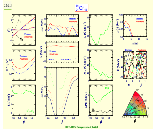
Chrome 66 (Z=24, N=42)
