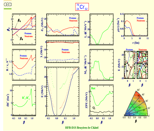
Chrome 76 (Z=24, N=52)
