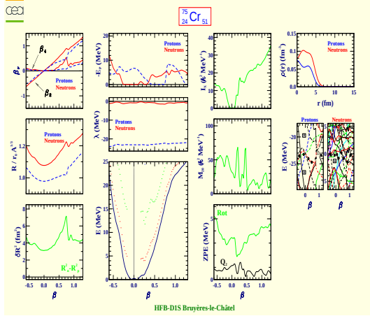
Chrome 75 (Z=24, N=51)
