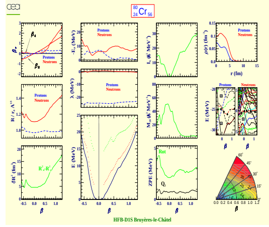
Chrome 80 (Z=24, N=56)
