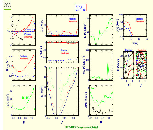
Vanadium 74 (Z=23, N=51)
