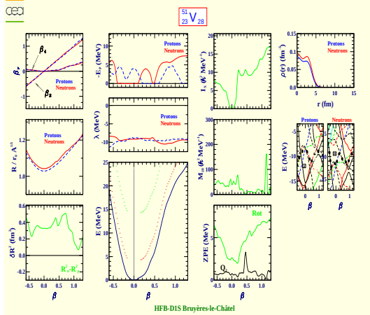
Vanadium 51 (Z=23, N=28)
