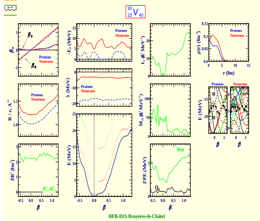
Vanadium 63 (Z=23, N=40)
