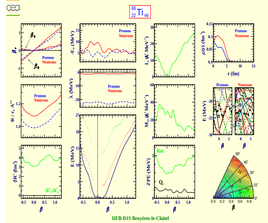
Titanium 68 (Z=22, N=46)
