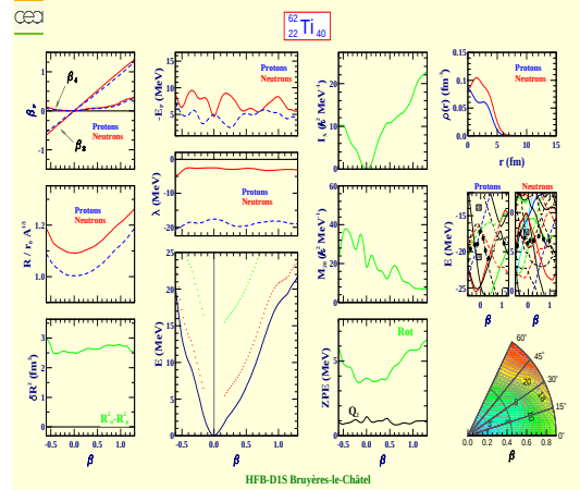
Titanium 62 (Z=22, N=40)
