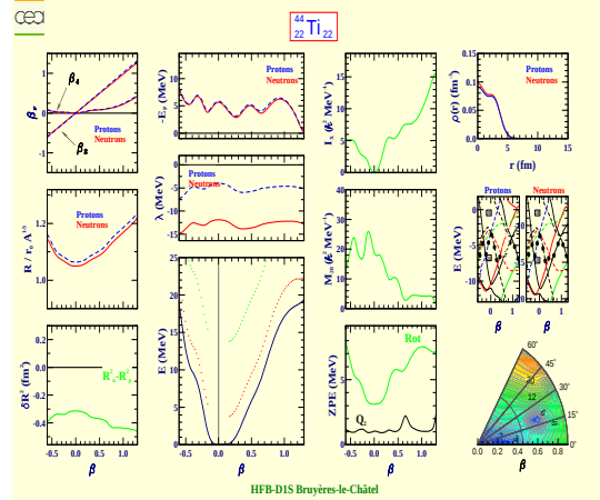
Titanium 44 (Z=22, N=22)
