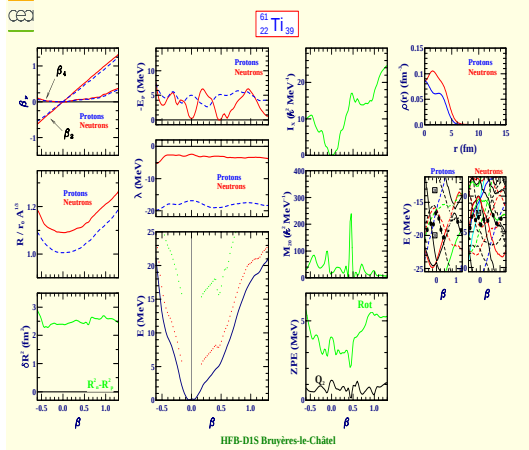
Titanium 61 (Z=22, N=39)
