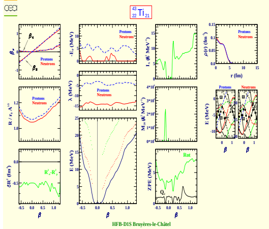
Titanium 43 (Z=22, N=21)
