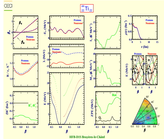
Titane 44 (Z=22, N=22)
