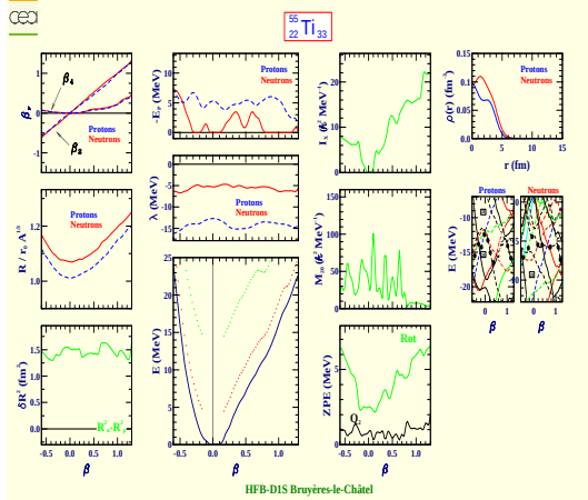
Titane 55 (Z=22, N=33)
