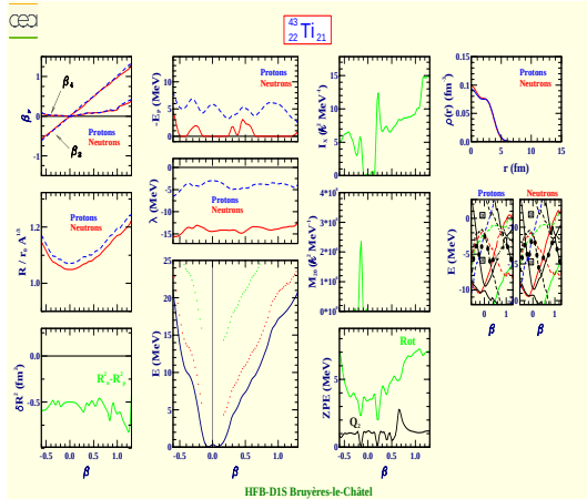
Titane 43 (Z=22, N=21)
