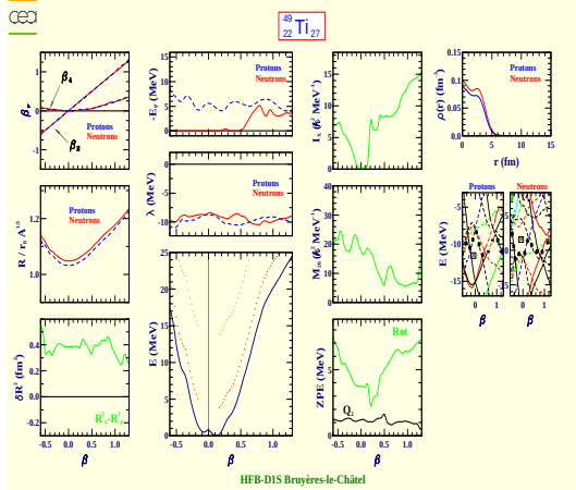
Titane 49 (Z=22, N=27)
