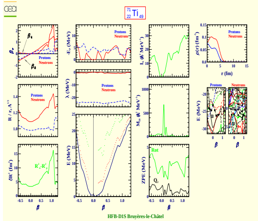
Titane 71 (Z=22, N=49)
