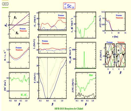
Scandium 47 (Z=21, N=26)
