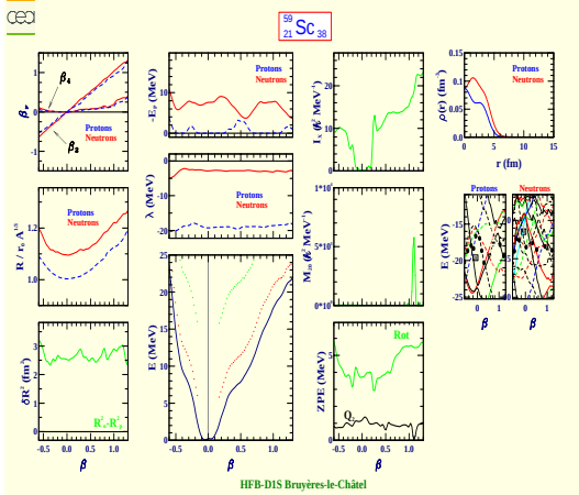
Scandium 59 (Z=21, N=38)
