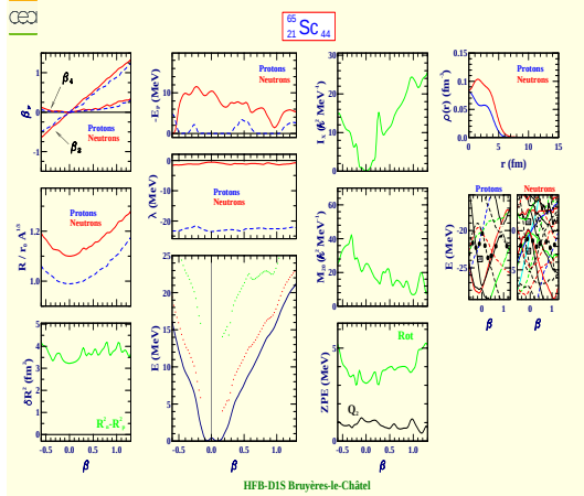
Scandium 65 (Z=21, N=44)
