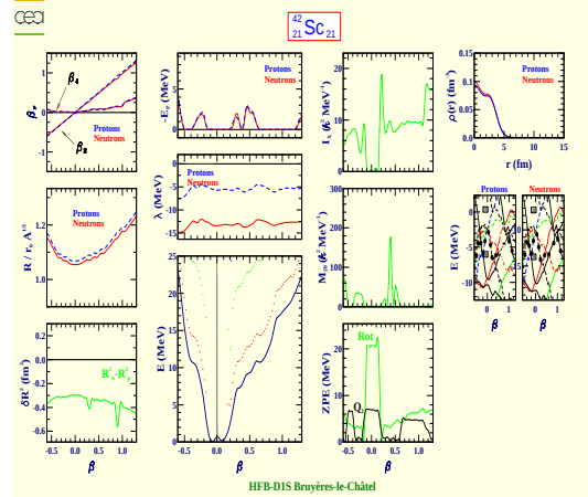
Scandium 42 (Z=21, N=21)
