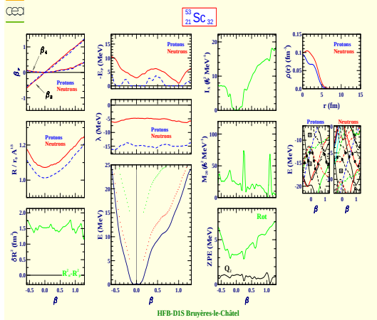
Scandium 53 (Z=21, N=32)
