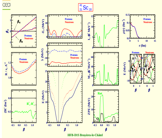
Scandium 41 (Z=21, N=20)
